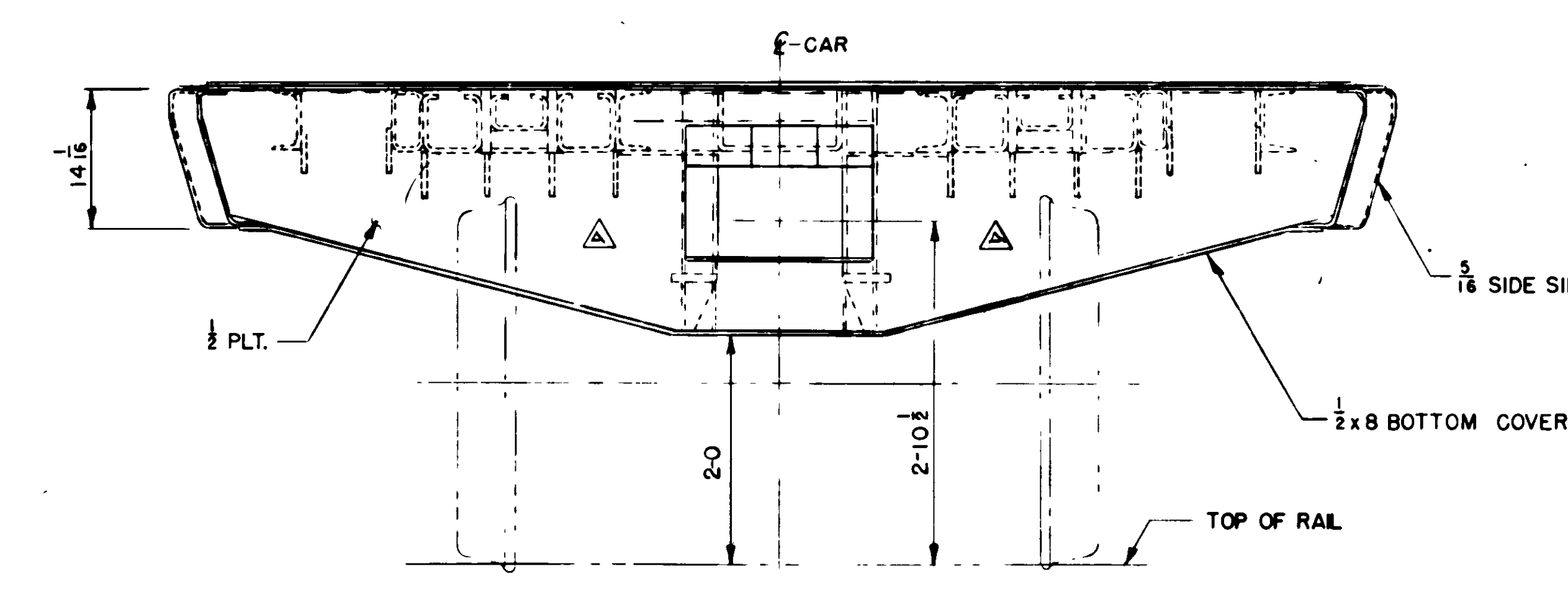
END VIEW SCALE: 1/4" = 1'-0"
