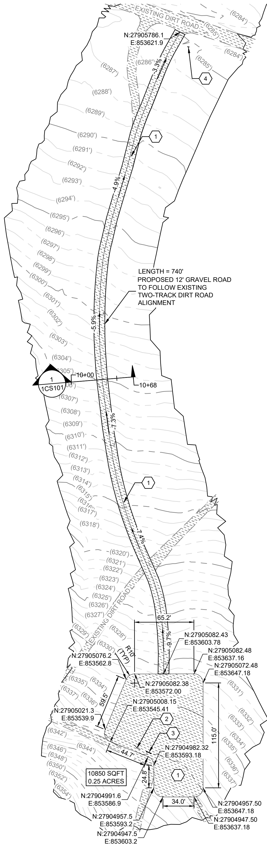
LACKAWANNA SITE PLAN
