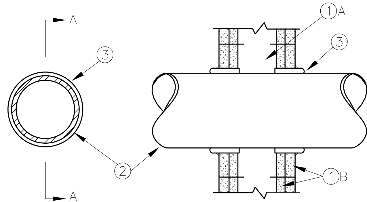
SECTION A-A
