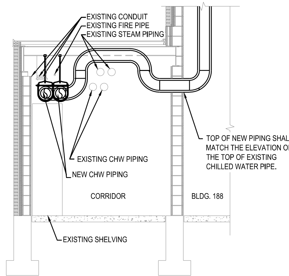
B9 CORRIDOR SECTION SCALE: 1/4" = 1'-0"
