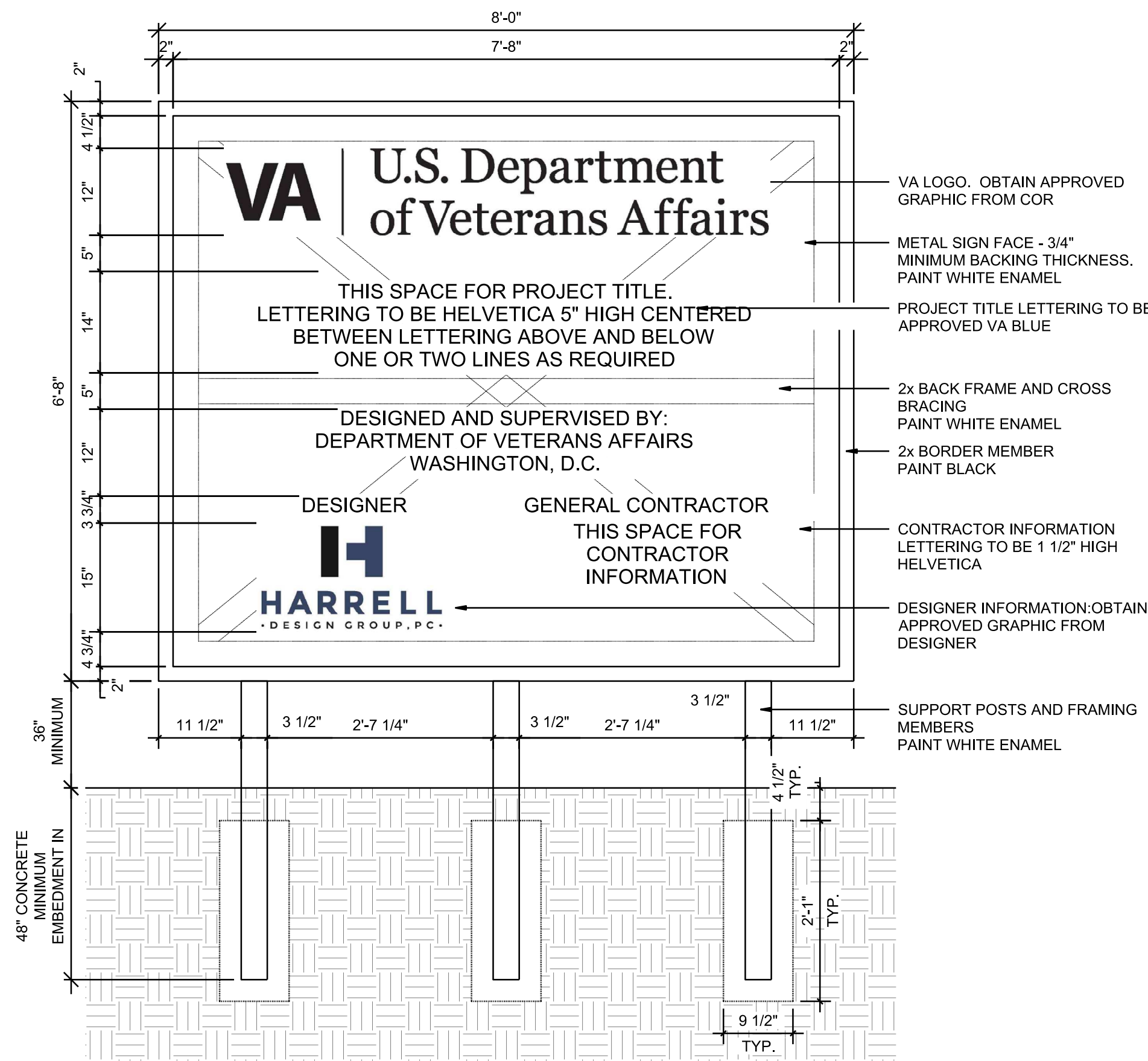
C1 PROJECT SIGN SCALE: 3/4" = 1'-0"
