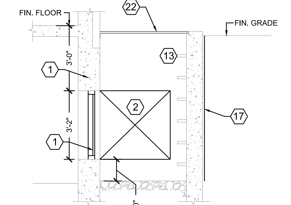
D8 SECTION SCALE: 3/8" = 1'-0"
