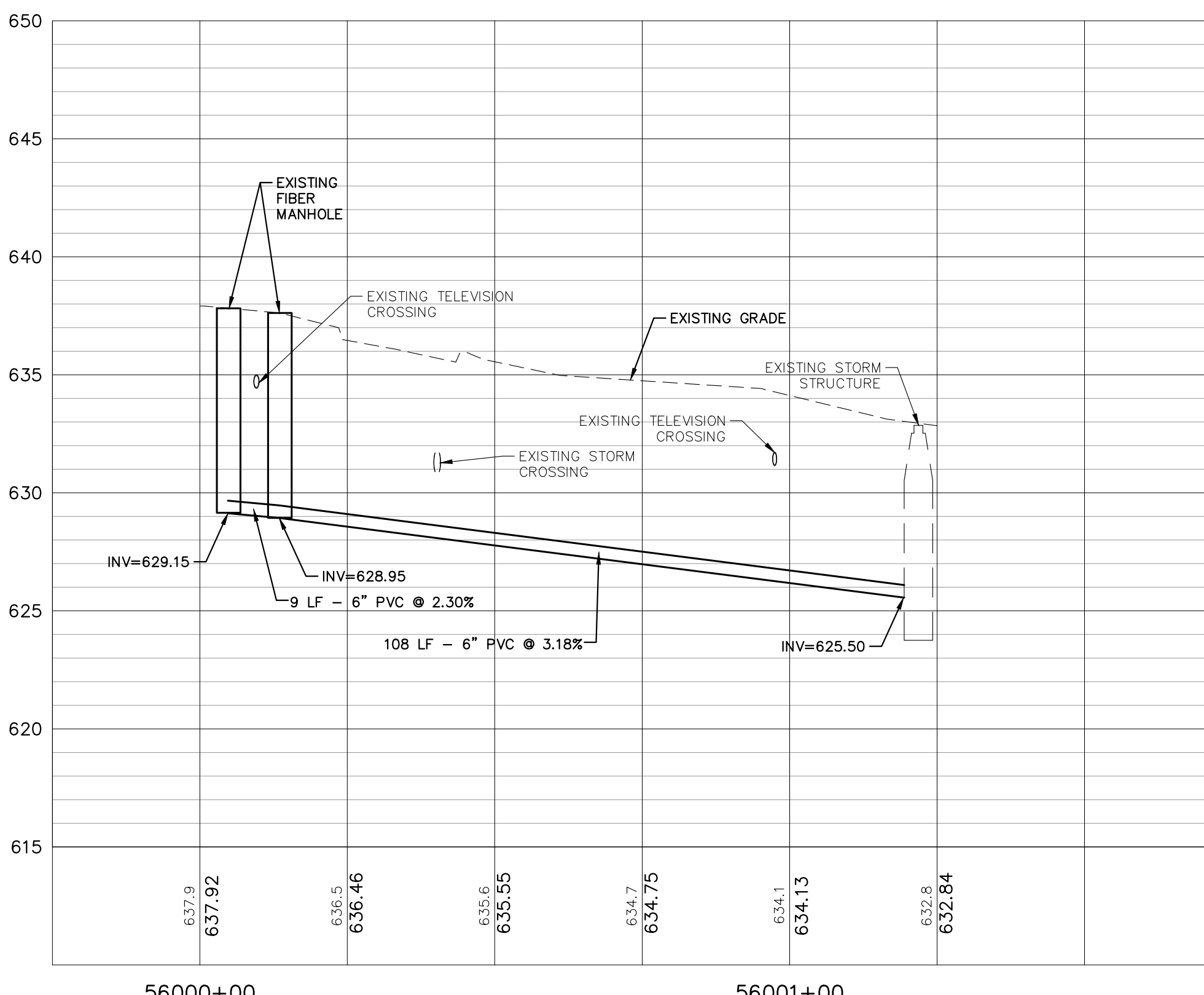
MANHOLE STORM 27
