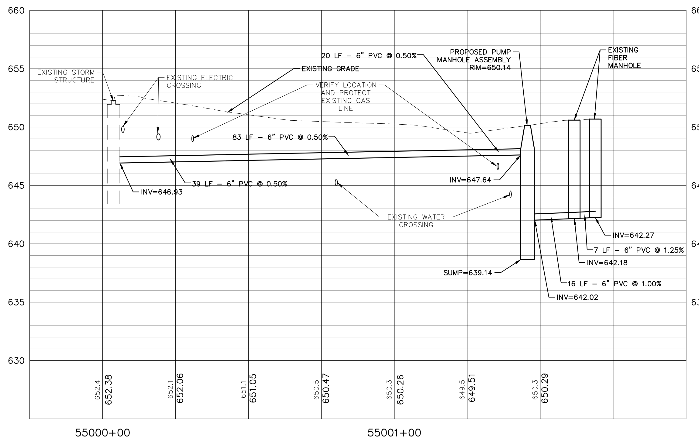
MANHOLE STORM 26
