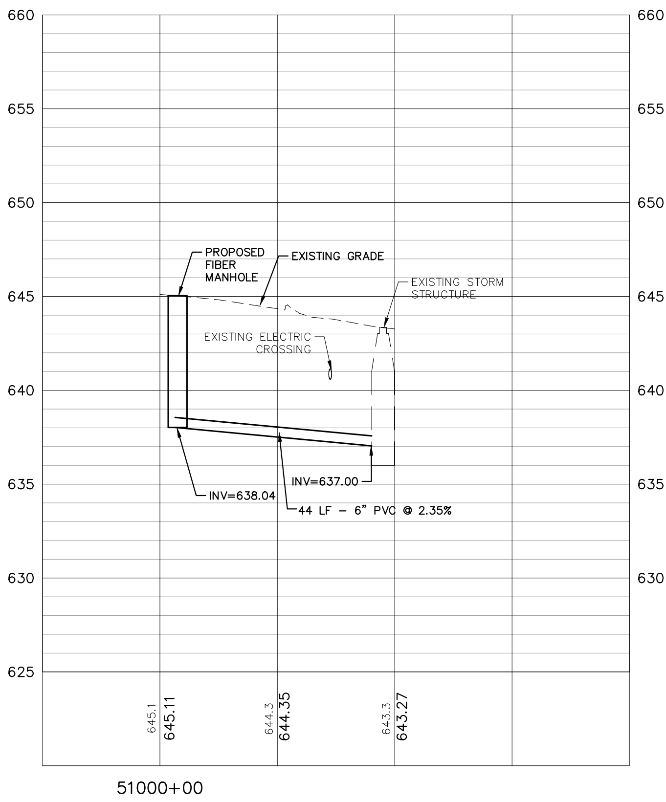
MANHOLE STORM 22
