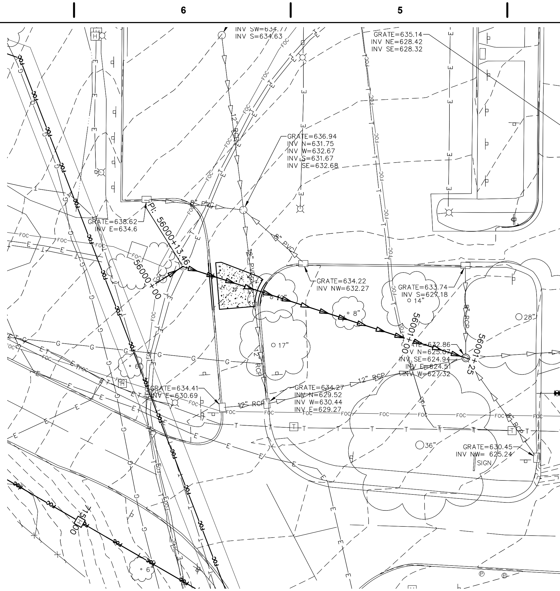
MANHOLE STORM 27 SCALE: 1"=20'
