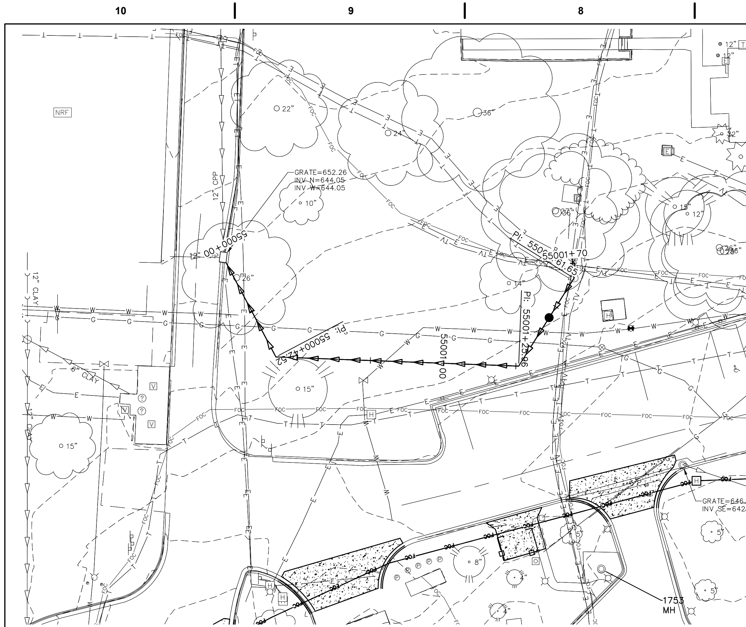
MANHOLE STORM 26 SCALE: 1"=20'
