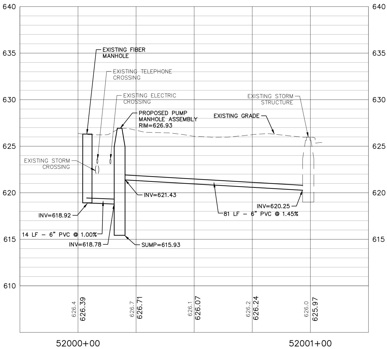
MANHOLE STORM 23
