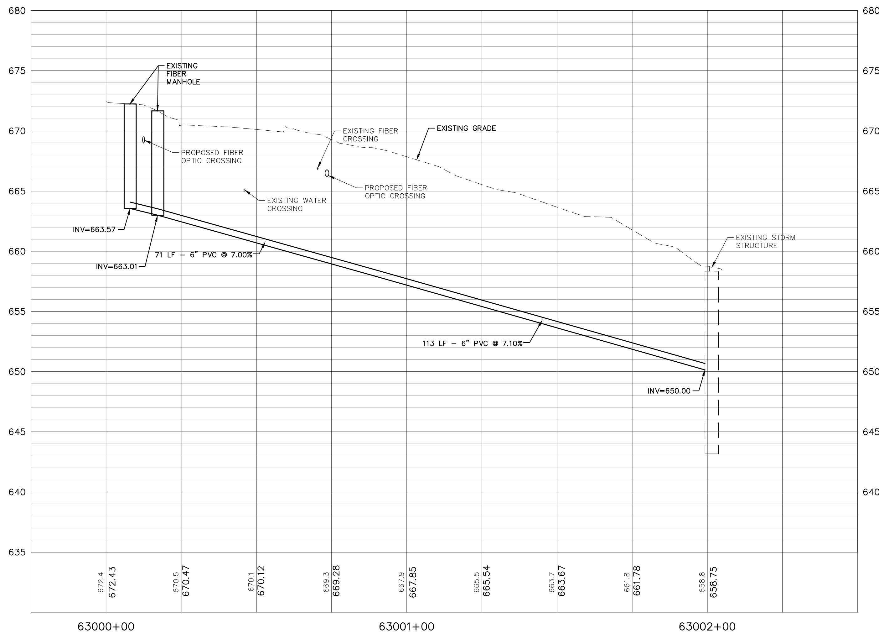
MANHOLE STORM 34
