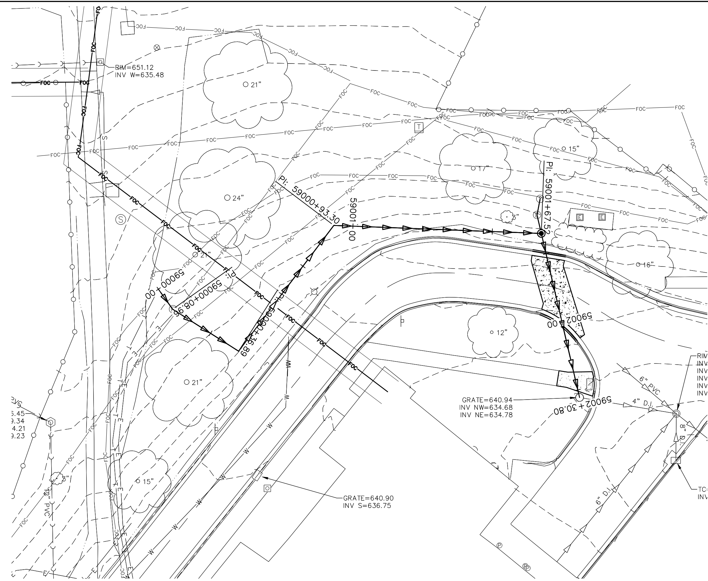
MANHOLE STORM 30 SCALE: 1"=20'
