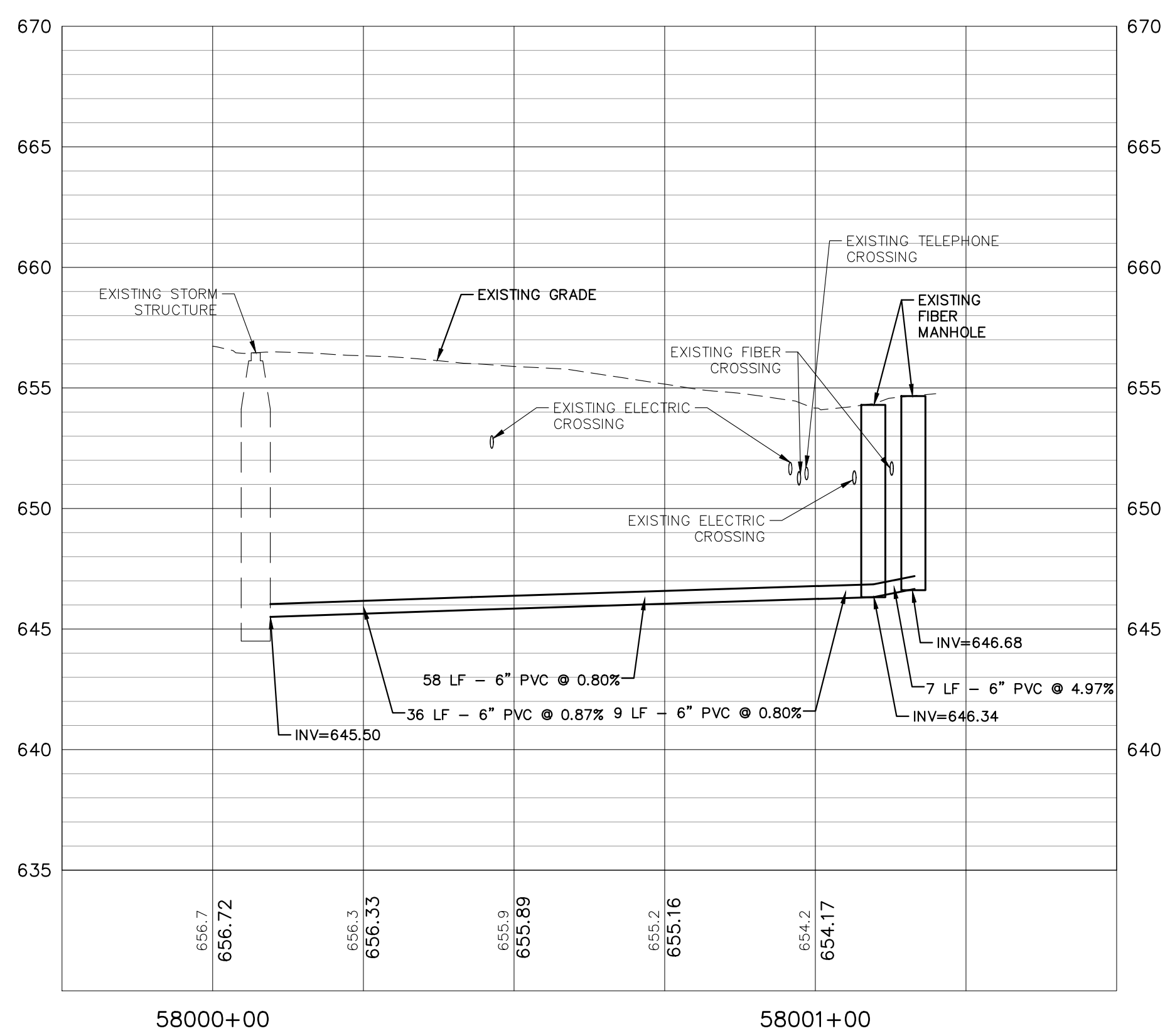
MANHOLE STORM 29
