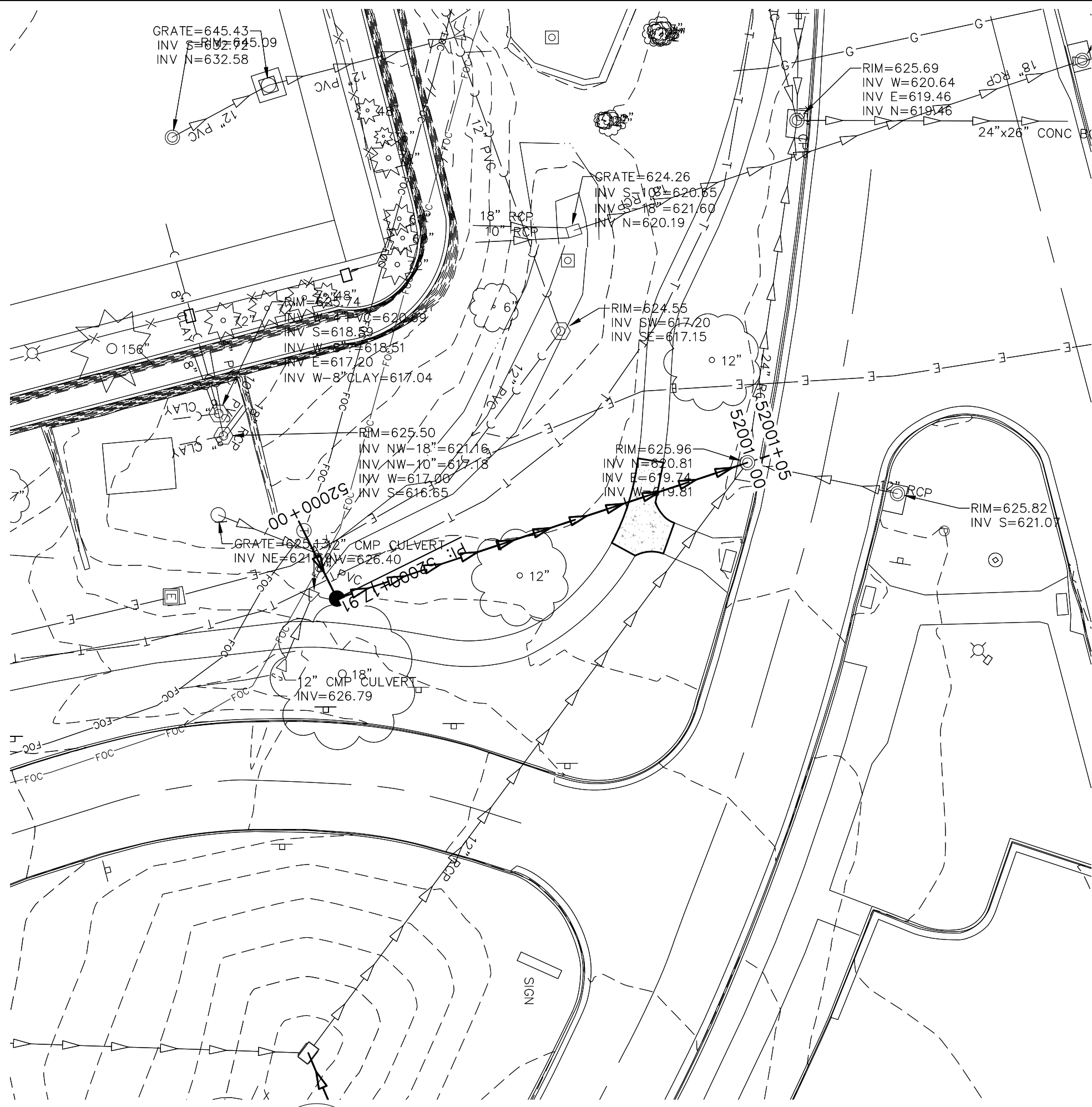
MANHOLE STORM 23 SCALE: 1"=20'
