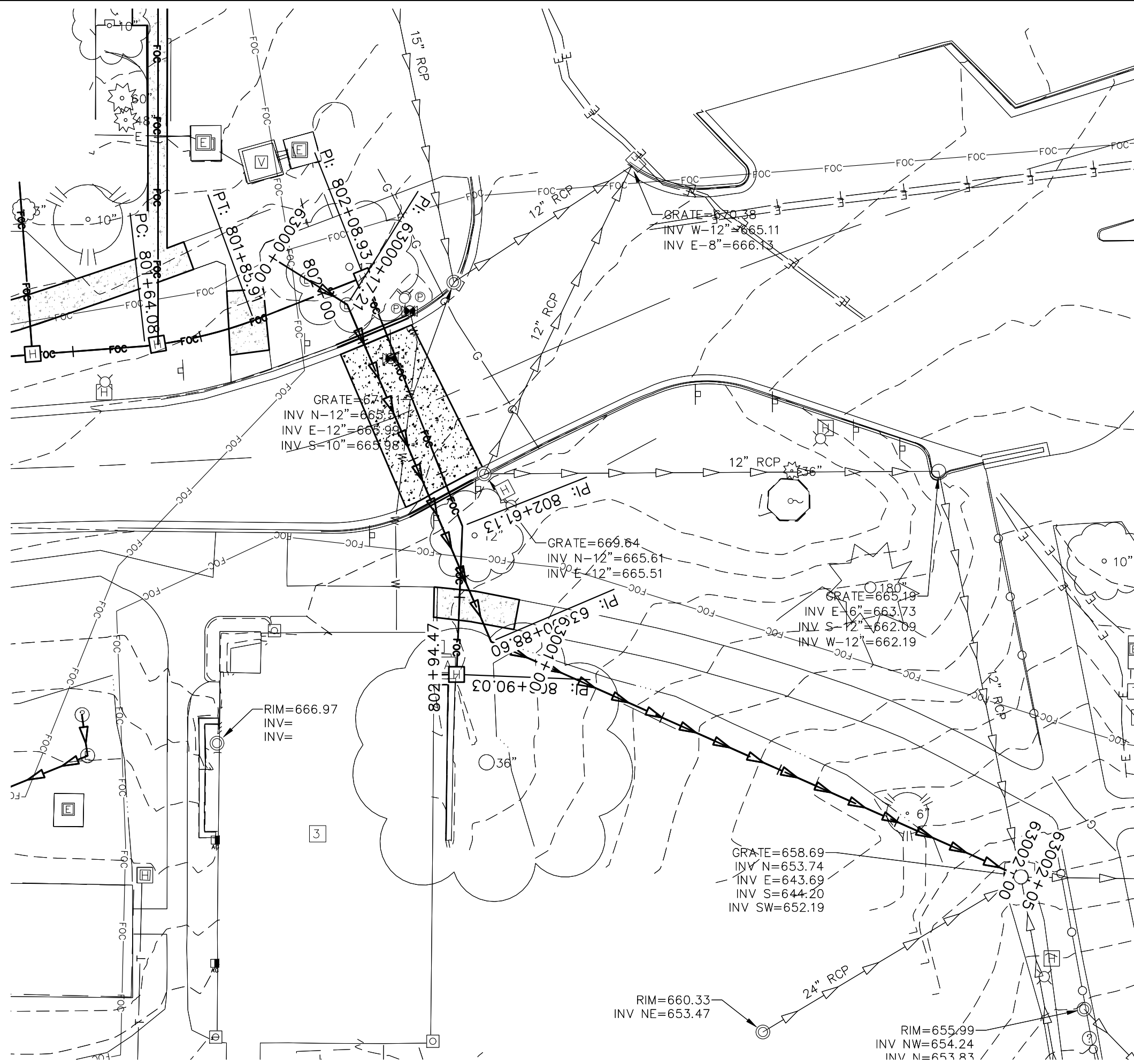
MANHOLE STORM 34 SCALE: 1"=20'
