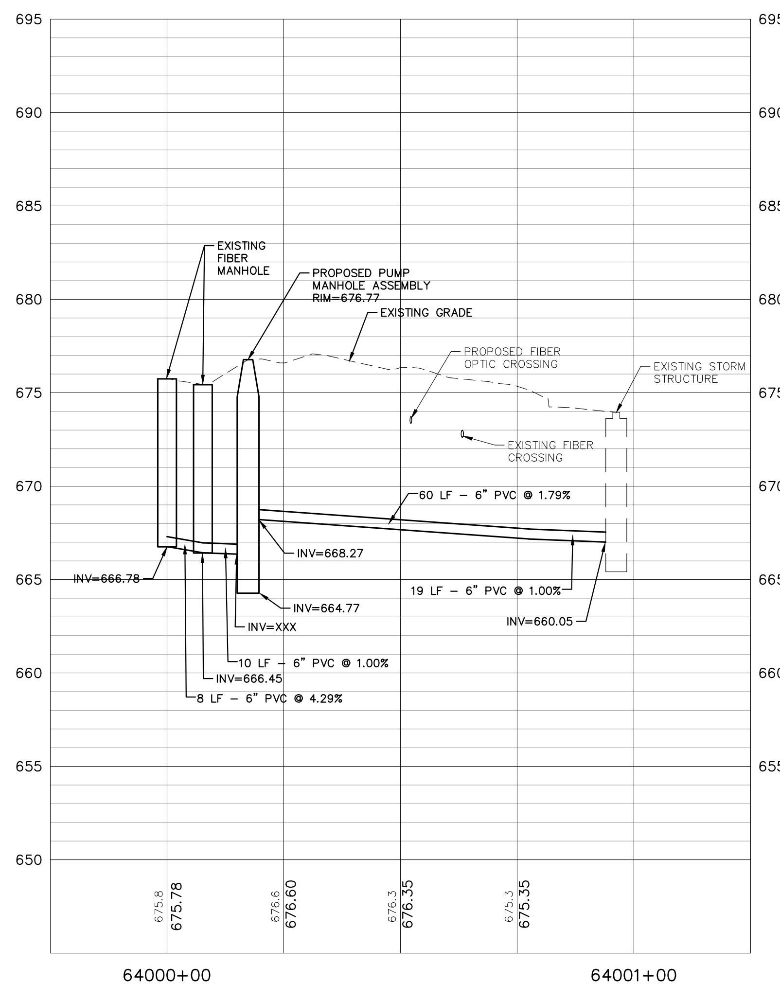
MANHOLE STORM 35
