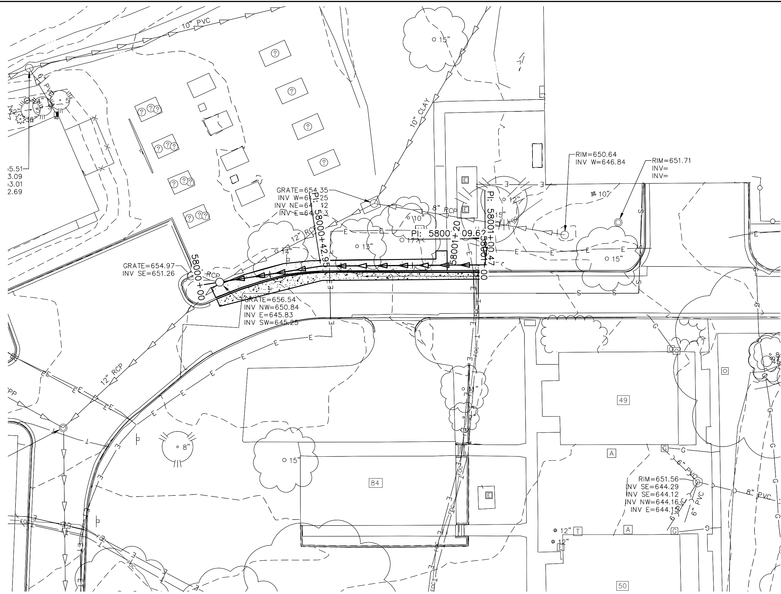
MANHOLE STORM 29 SCALE: 1"=20'
