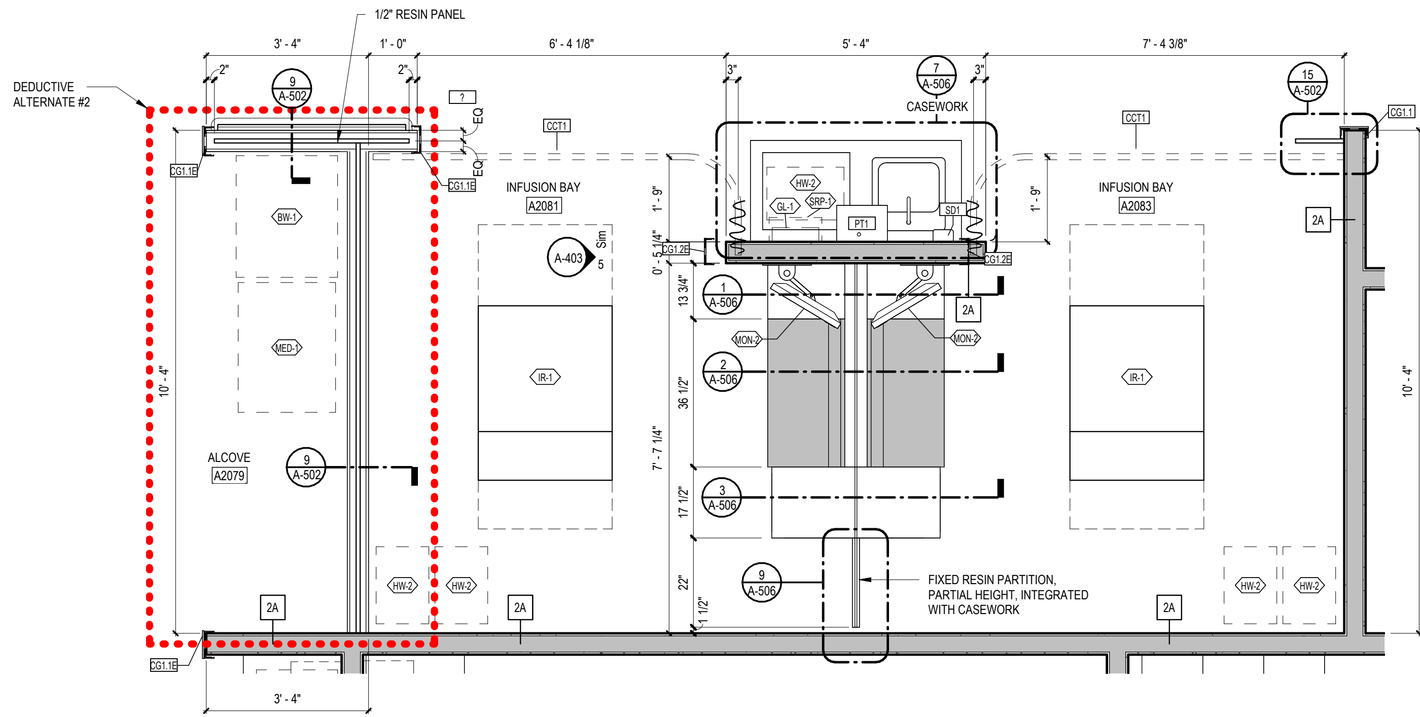
8 INFUSION BAY - A2081 A2083
