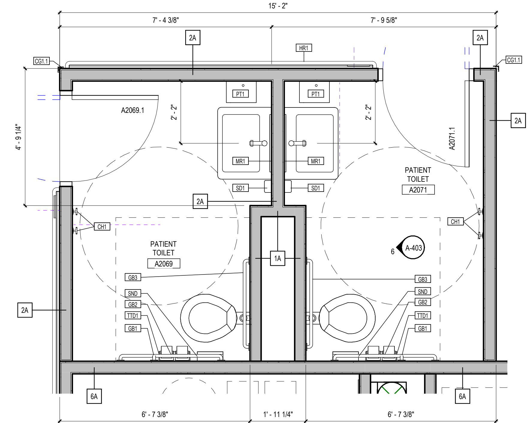
1 PATIENT TOILET - A2069 & A2071
