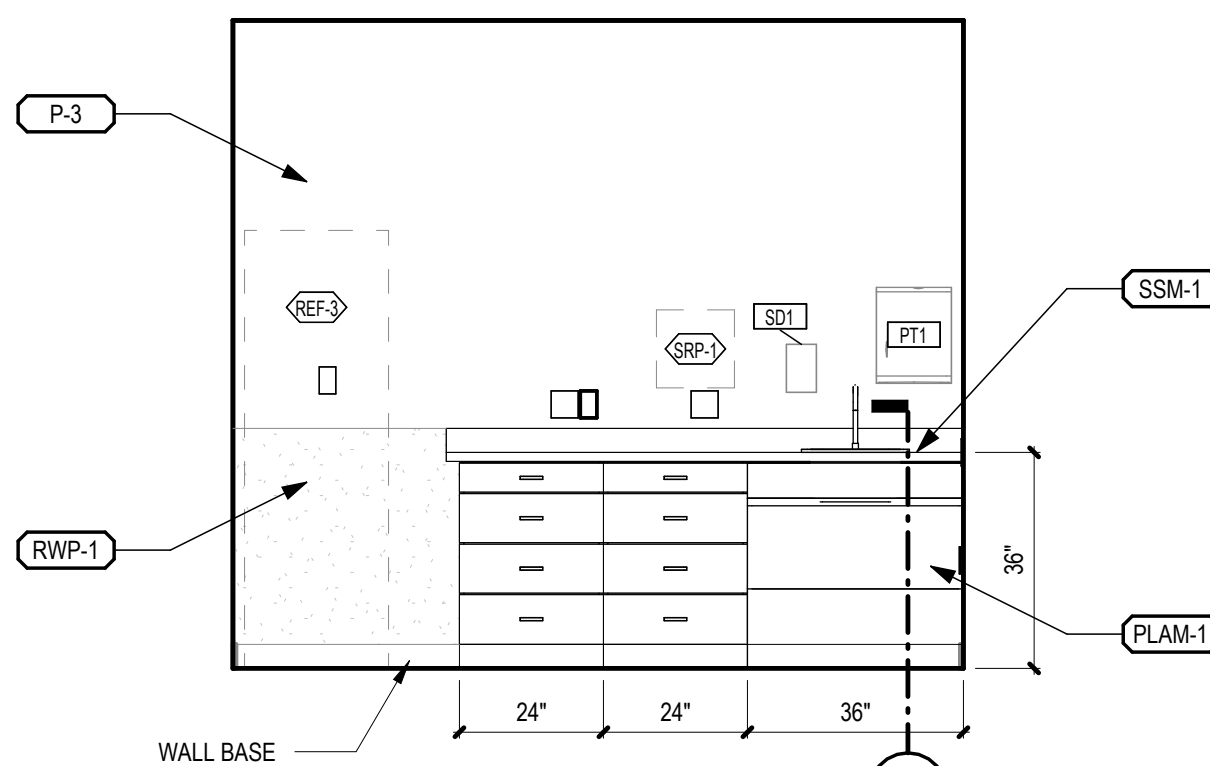
15 MED ROOM A2046 - WEST A-102.1C 3/8" = 1'-0"
