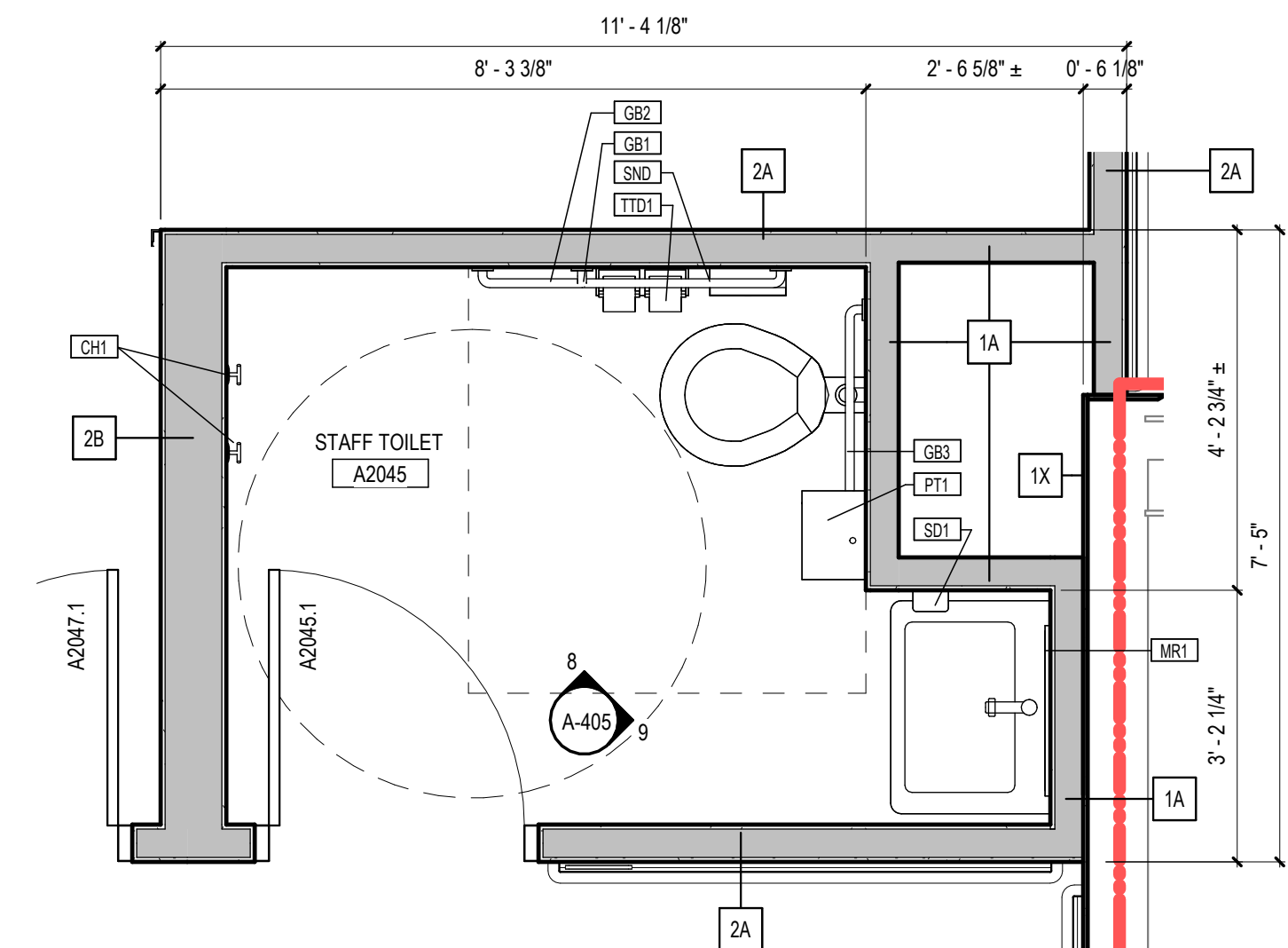
5 STAFF TOILET - A2045
