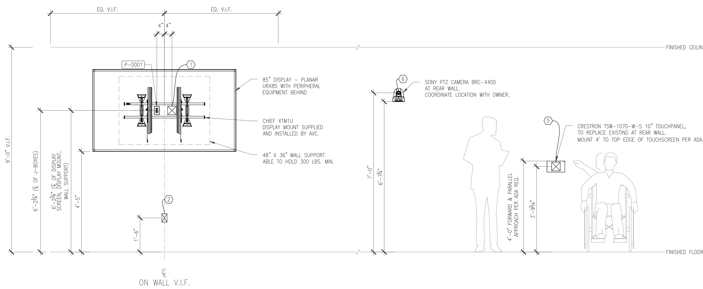
B CLASSROOM 1A, 2A, 3A - AV EQUIPMENT ELEVATION SCALE: 1/2" = 1'-0"
