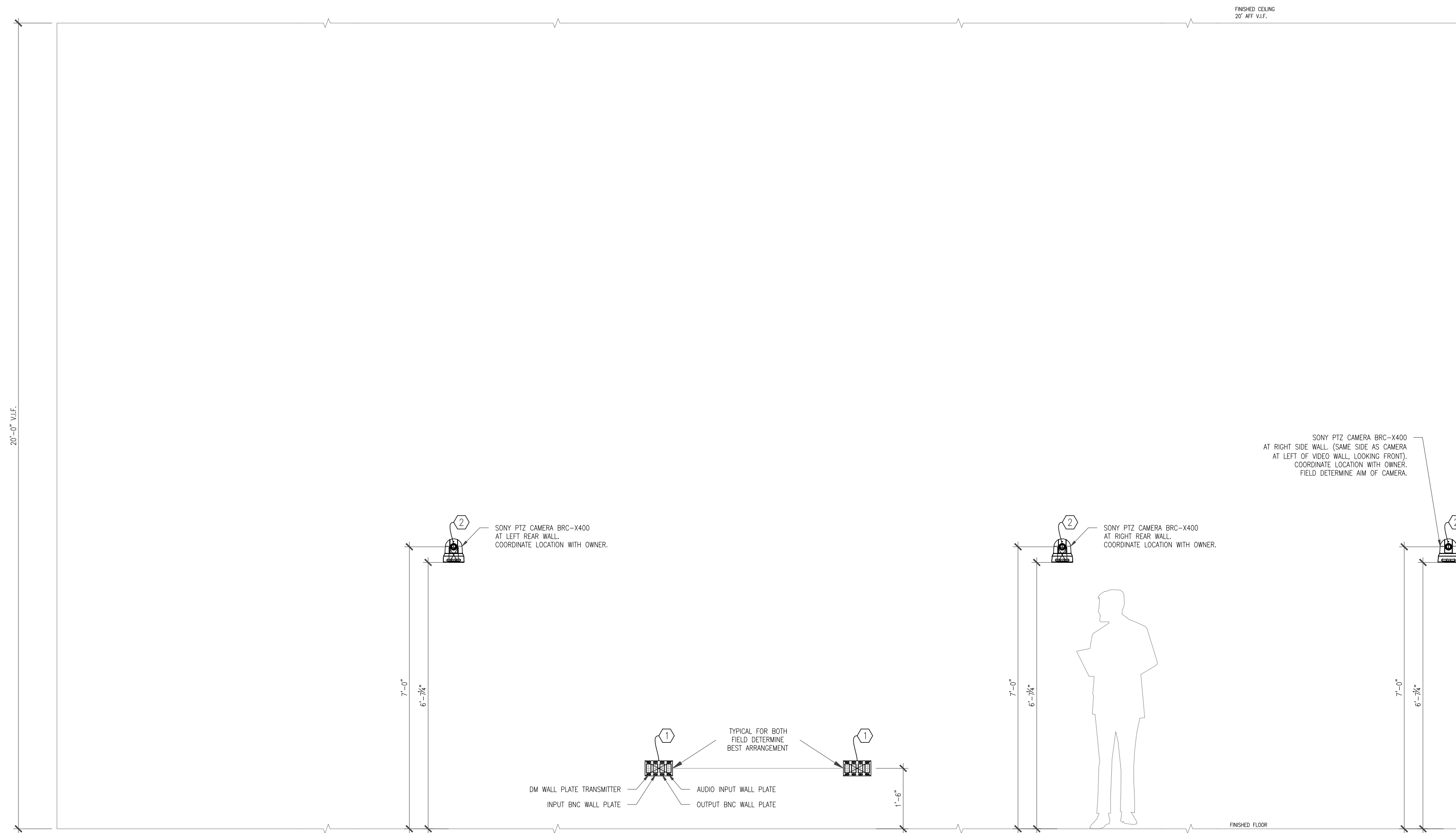
A AUDITORIUM AV EQUIPMENT ELEVATION SCALE: 1/2" = 1'-0"
