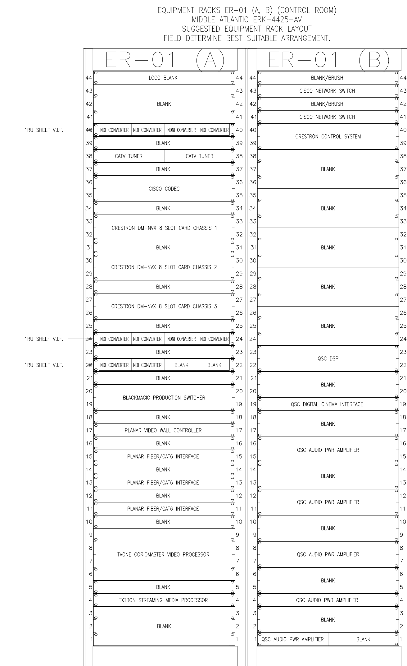
E CONTROL ROOM - AV EQUIPMENT RACKS ELEVATION SCALE: 1-1/2" = 1'-0"
