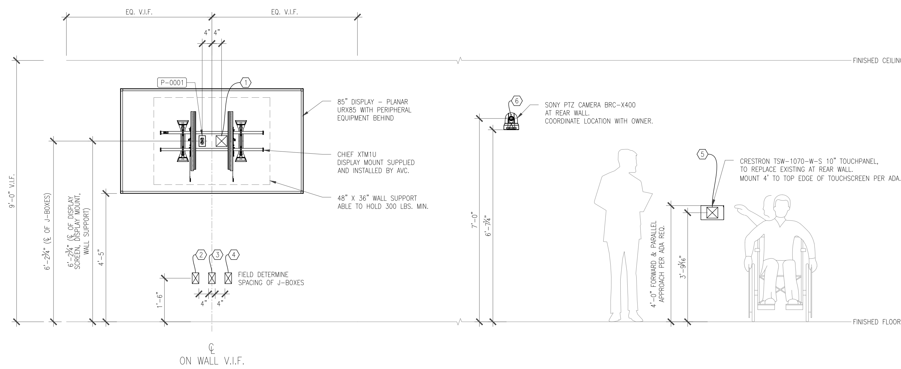
C CLASSROOM 1B, 2B, 3B - AV EQUIPMENT ELEVATION SCALE: 1/2" = 1'-0"
