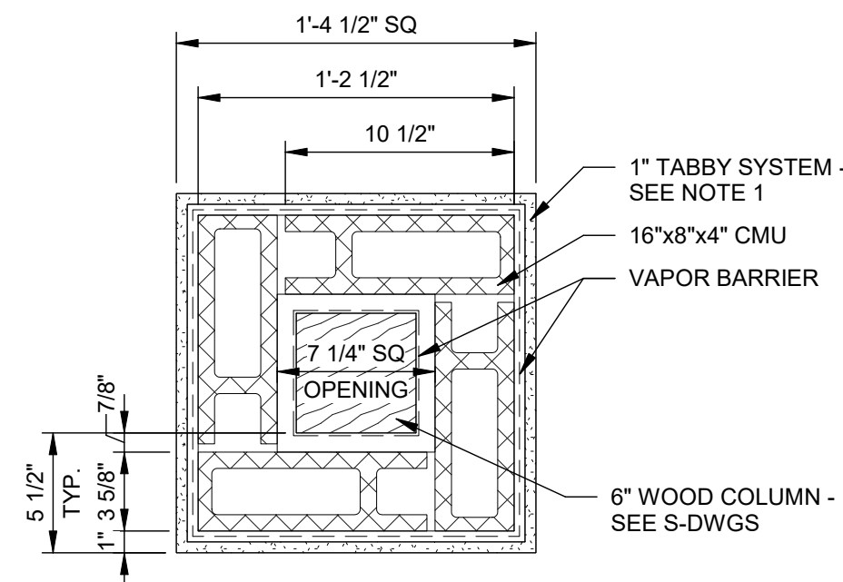
6 COLUMN BASE A-904 SCALE: 1 1/2" = 1'-0"
