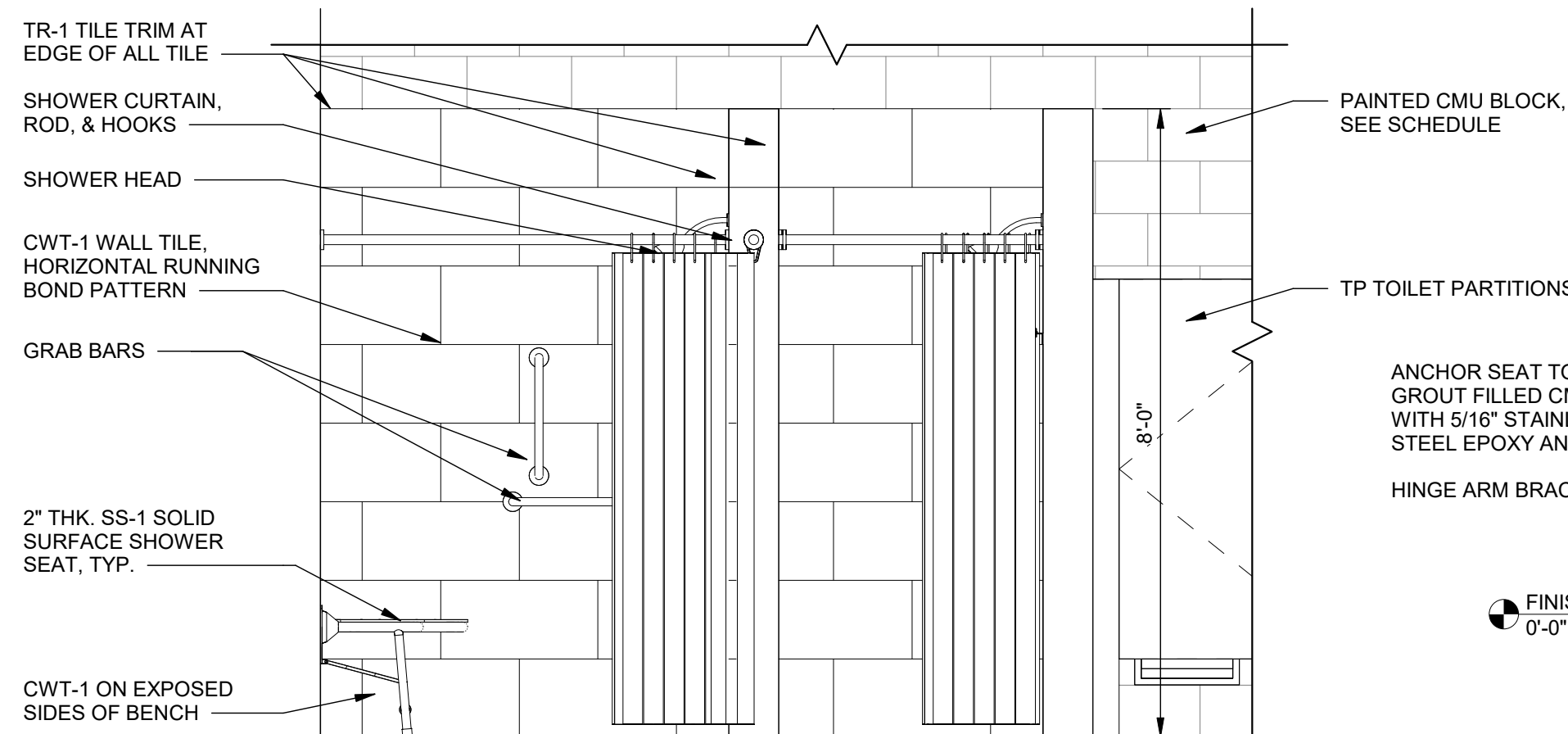
6 ELEVATION - SHOWERS A-902 SCALE: 1/2" = 1'-0"
