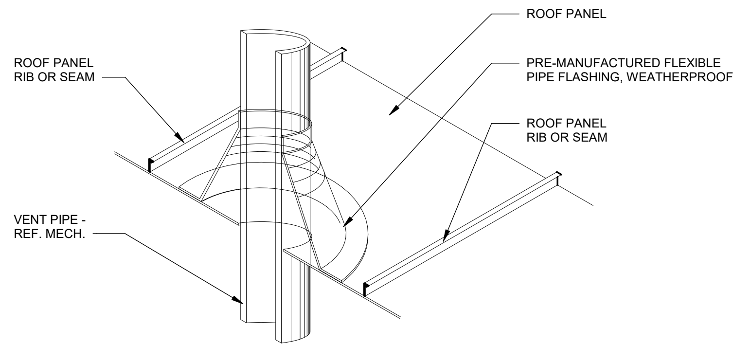
2 VTR PIPE PENETRATION A-905 SCALE: 1 1/2" = 1'-0"
