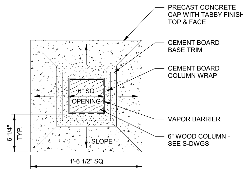
5 COLUMN @ PRECAST CAP A-904 SCALE: 1 1/2" = 1'-0"
