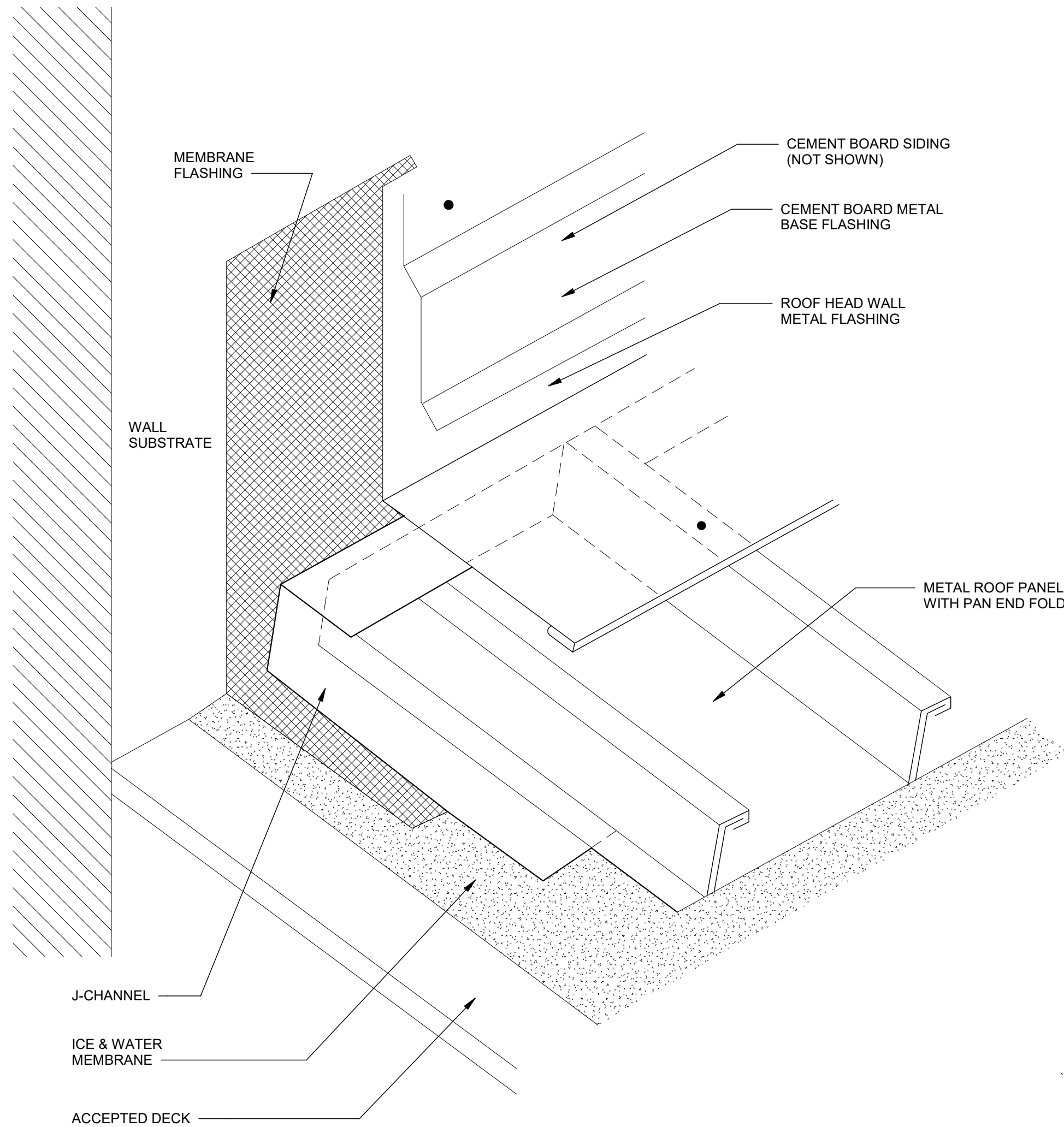
1 HEADWALL DETAIL A-905 SCALE: 3" = 1'-0"
