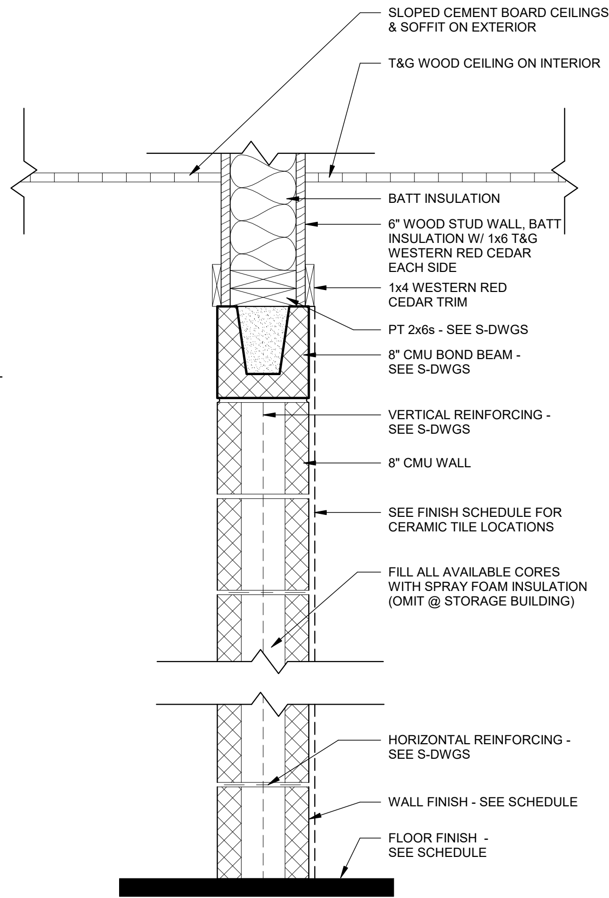
2 WALL TYPE 2 A-904 SCALE: 1 1/2" = 1'-0"
