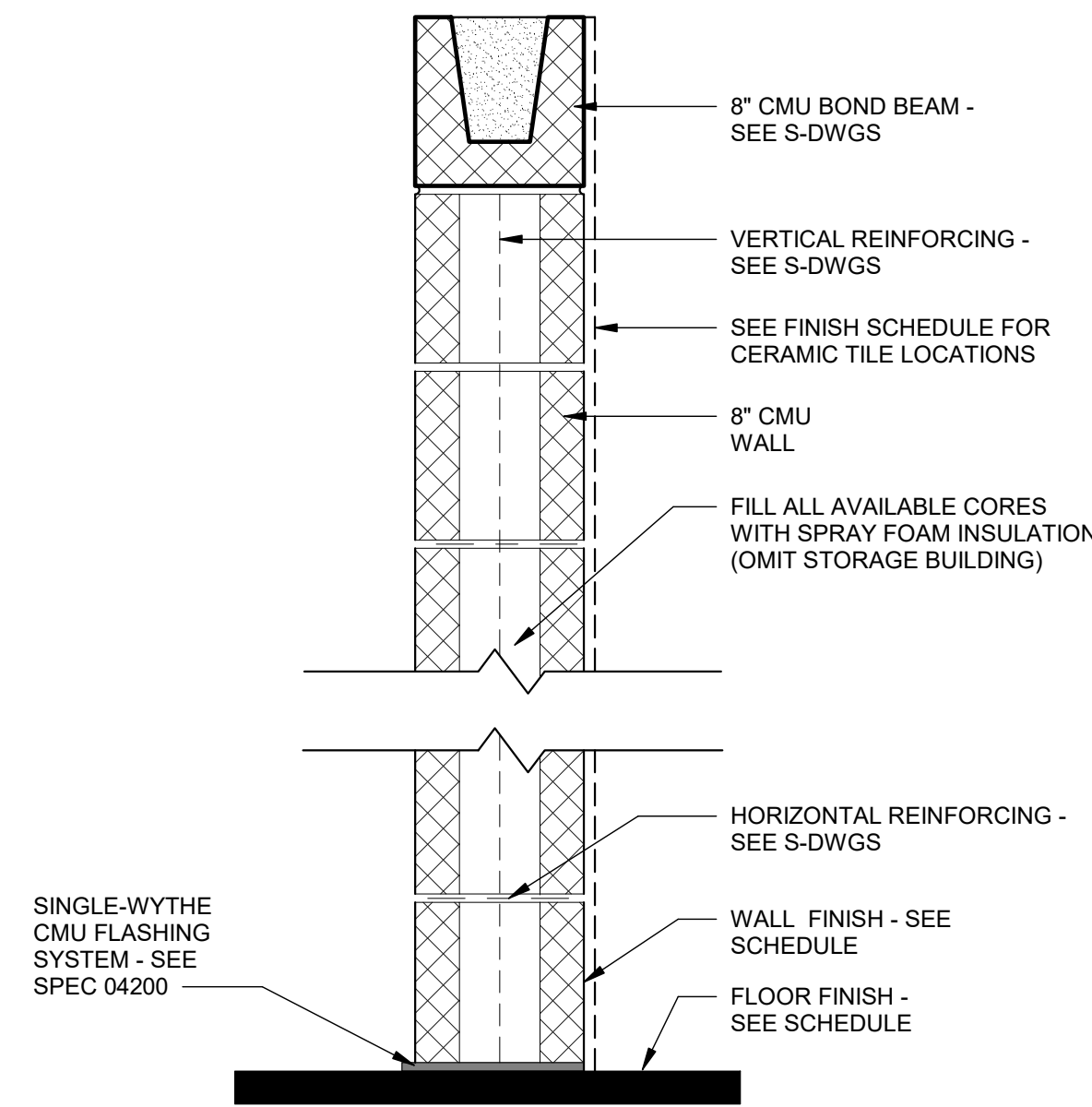
3 WALL TYPE 3 A-904 SCALE: 1 1/2" = 1'-0"
