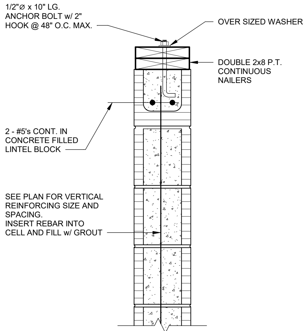
SECTION SCALE: 1 1/2" = 1'-0"
