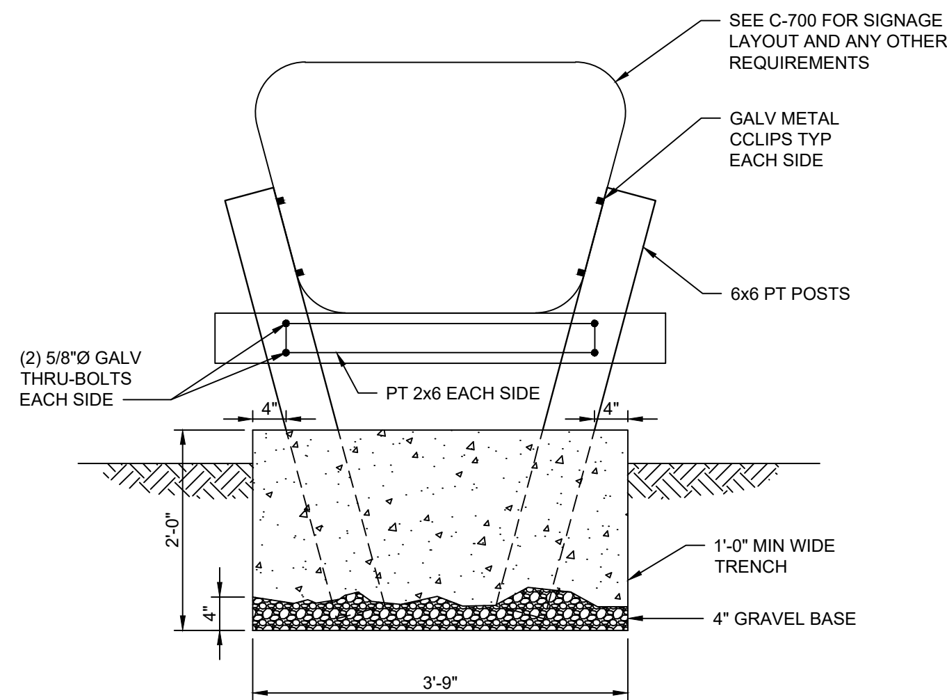
2 SITE SIGN 2 S-602 SCALE: 3/4"=1'-0"
