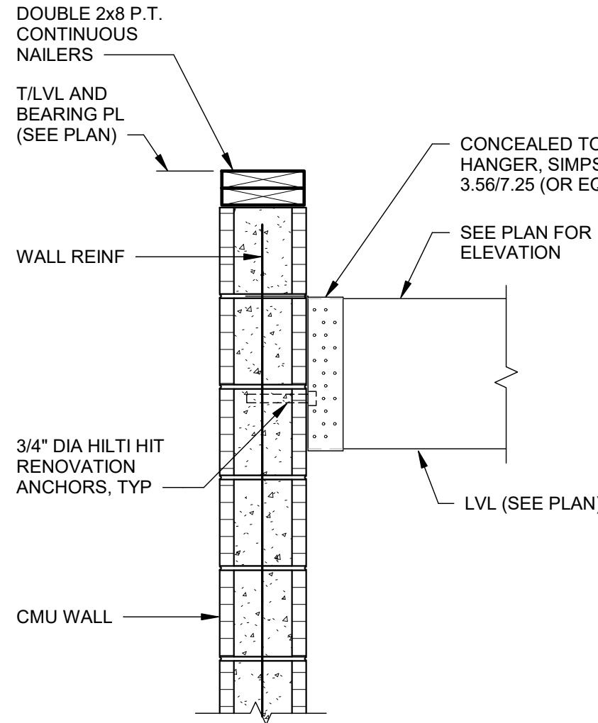
SECTION SCALE: 1" = 1'-0"
