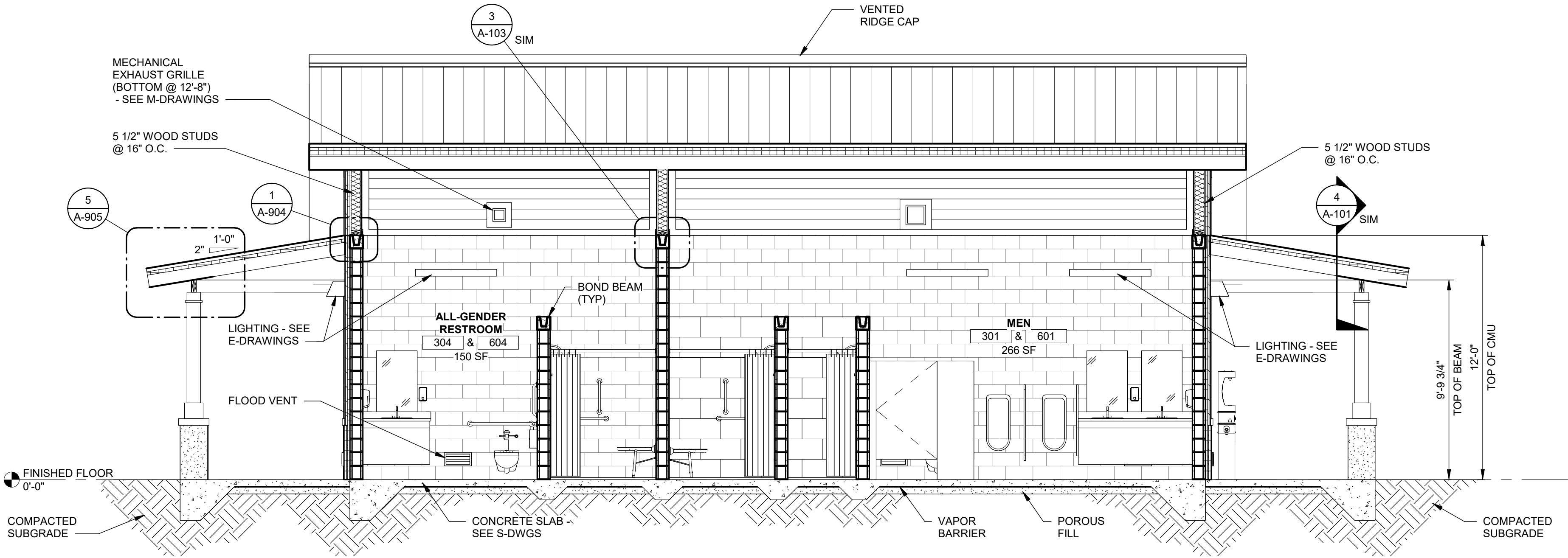
1 BUILDINGS 300/600 - LONGITUDINAL SECTION A-303 SCALE: 1/4" = 1'-0"
