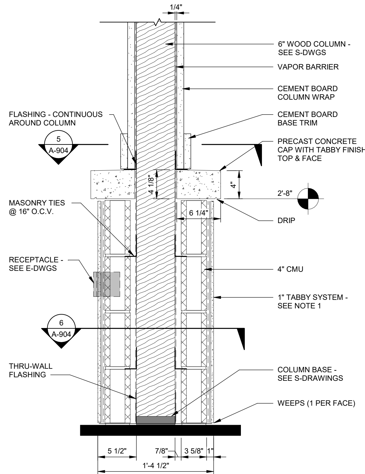
4 COLUMN SECTION A-904 SCALE: 1 1/2" = 1'-0"
