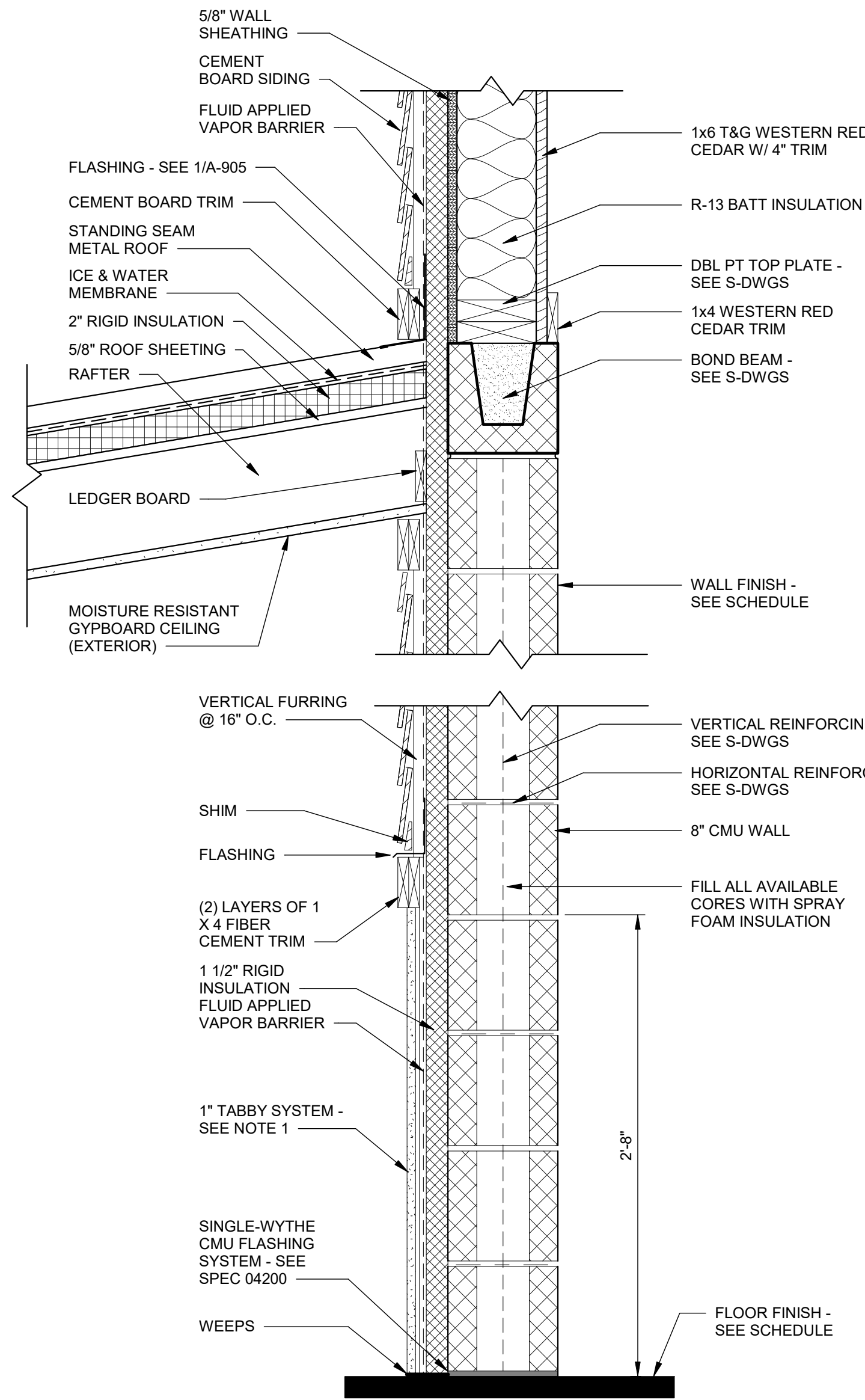
1 WALL TYPE 1 A-904 SCALE: 1 1/2" = 1'-0"
