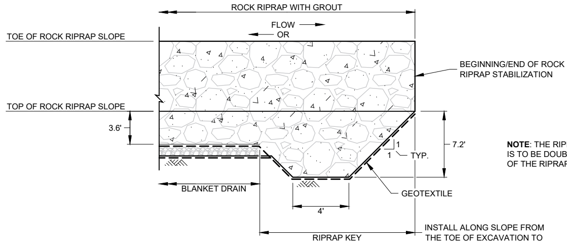
PLAN - RIPRAP KEY
