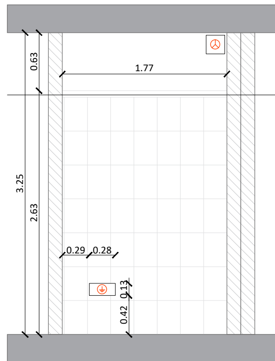
EL 2 EXISTING SCALE 1 : 40
