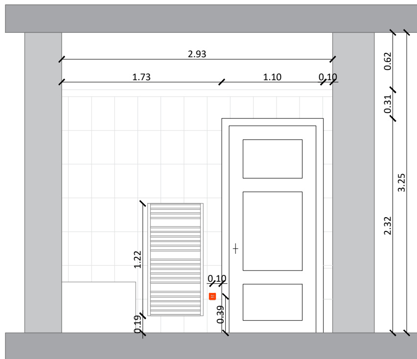
EL 3 EXISTING SCALE 1 : 40
