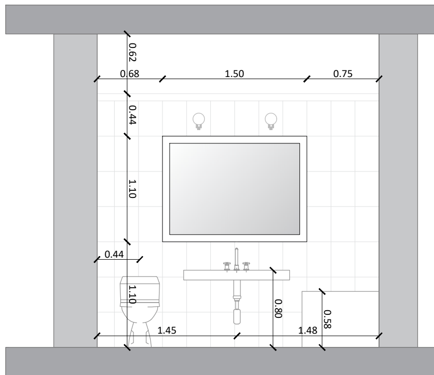
EL 1 EXISTING SCALE 1 : 40
