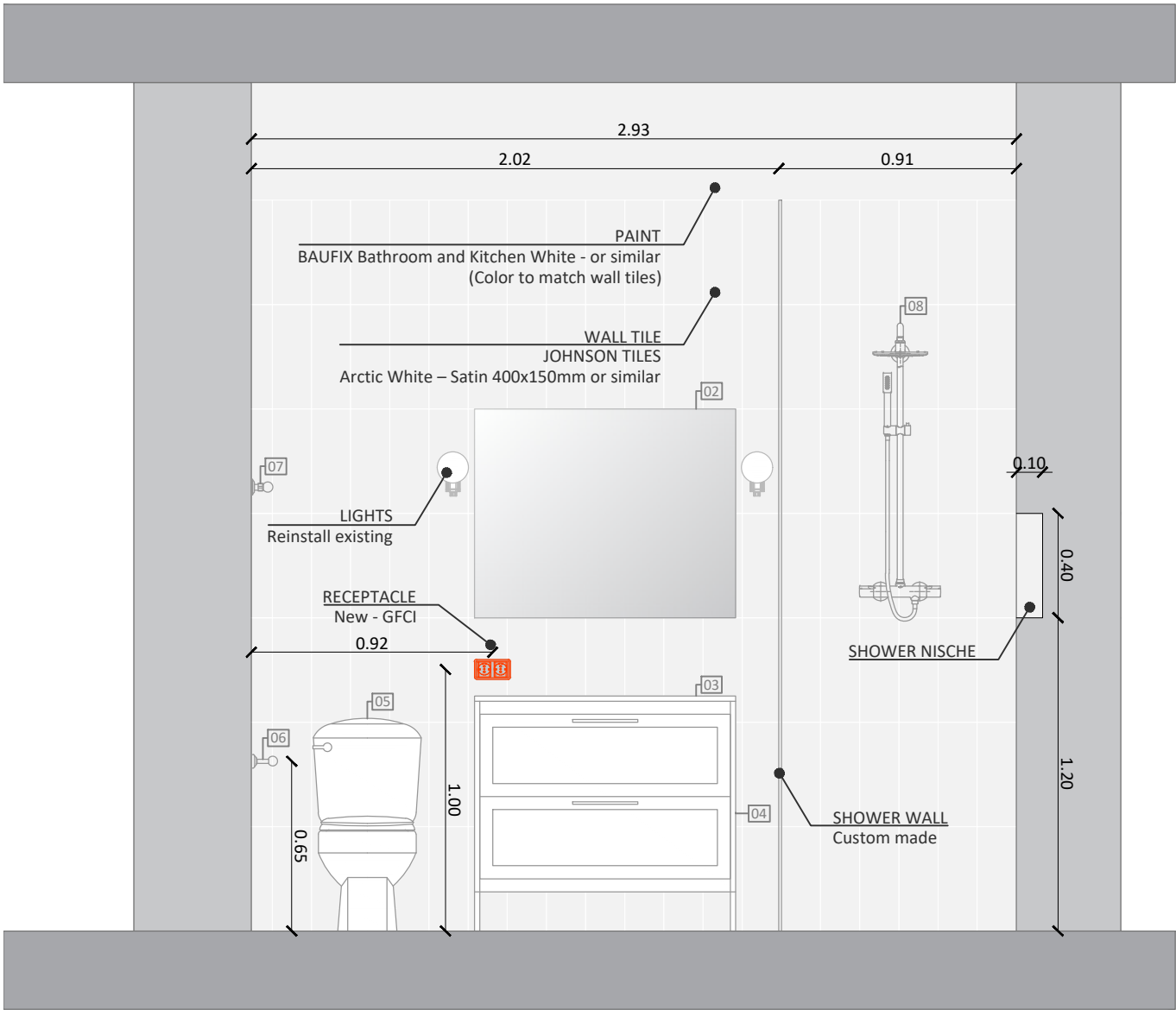
EL 1 NEW BATHROOM SCALE 1 : 25
