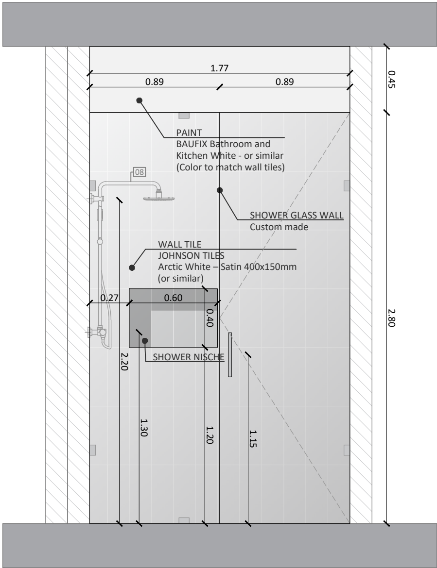
EL 2 NEW BATHROOM SCALE 1 : 25
