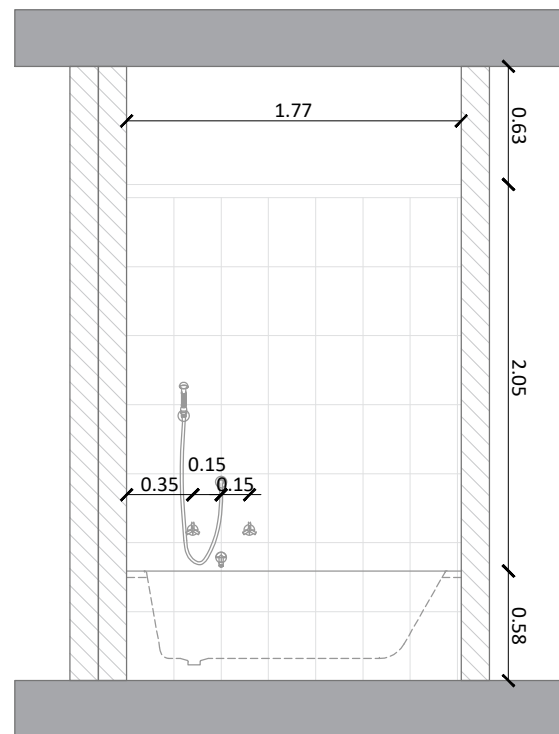
EL 4 EXISTING SCALE 1 : 40
