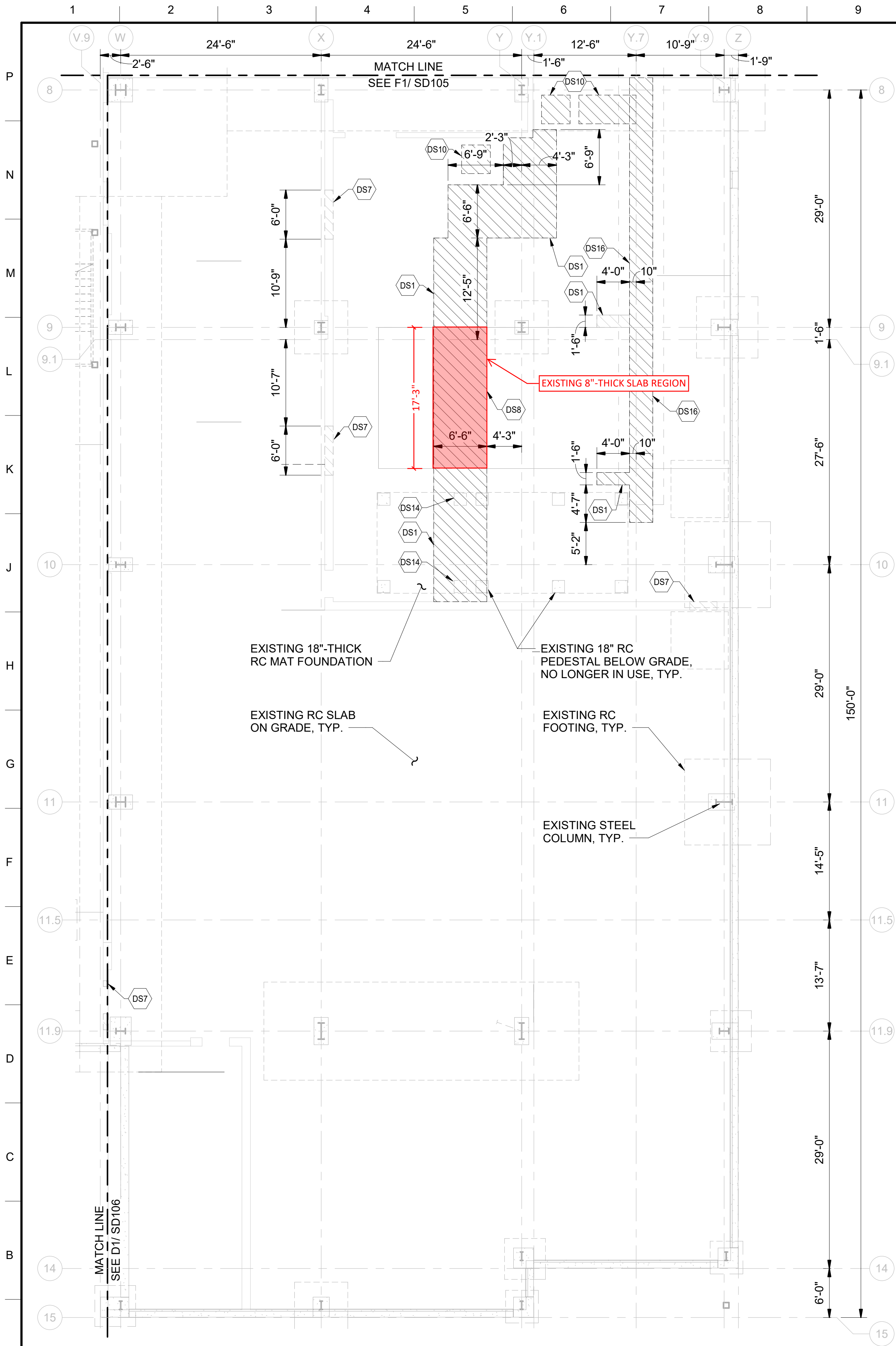
A1 FOUNDATION DEMOLITION PLAN - AREA D8 SCALE: 1/8" = 1'-0"
