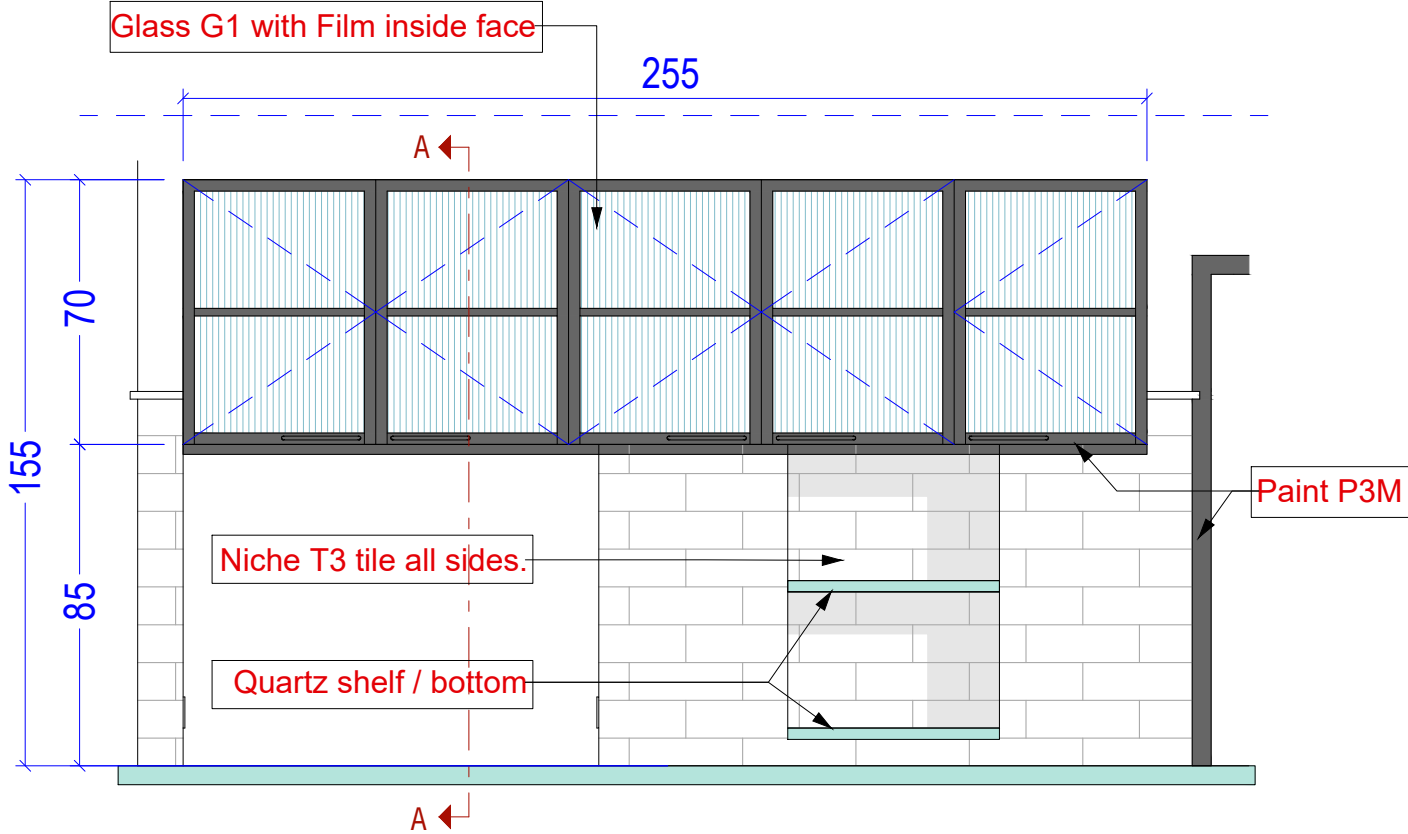
ELEVATION
