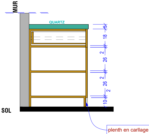
COUPE -AA-
