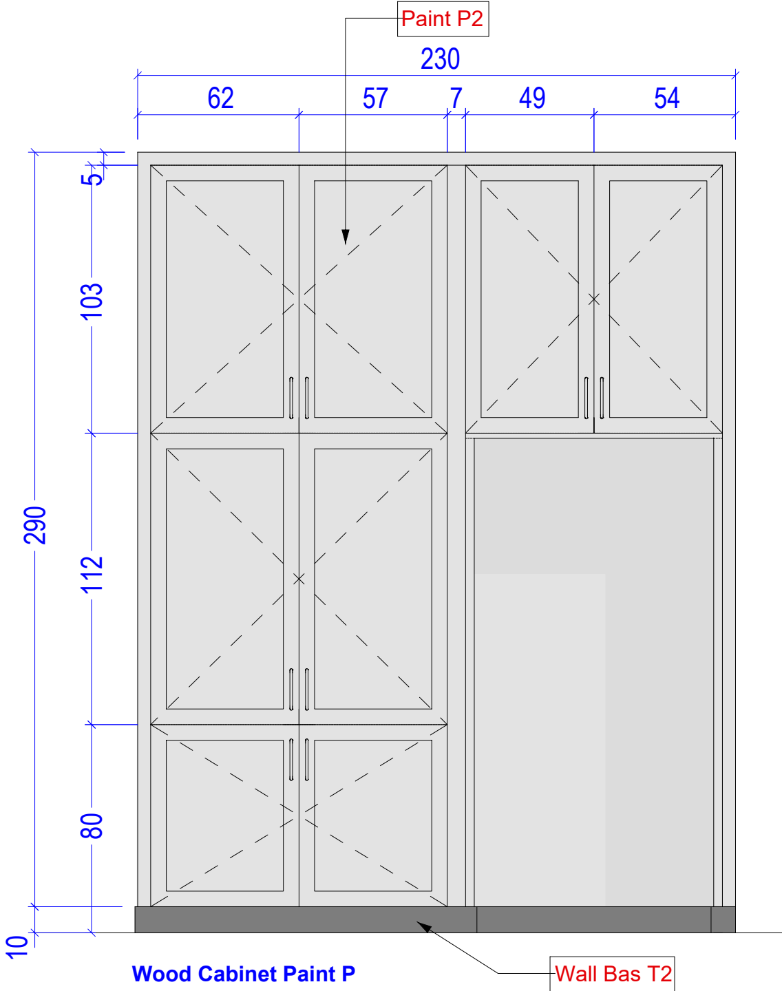
ELEVATION EXTERIEUR
