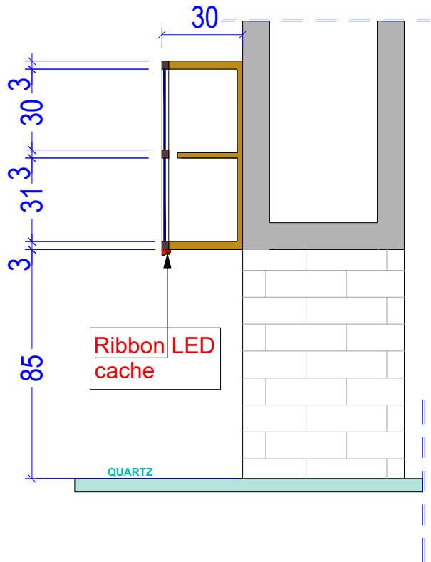
COUPE -AA-
