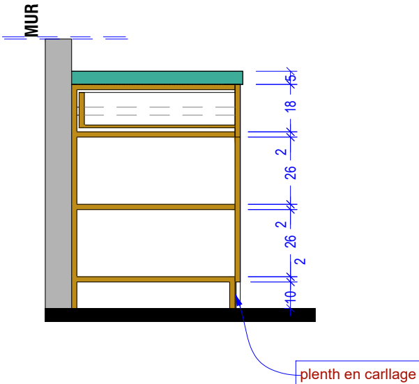
COUPE -AA-
