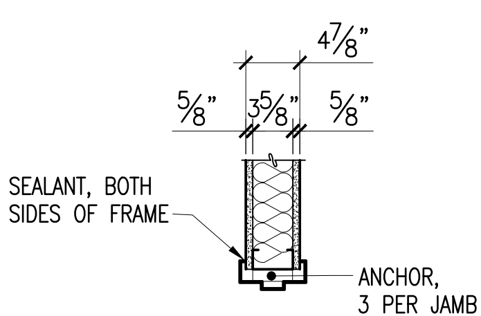
A JAMB
