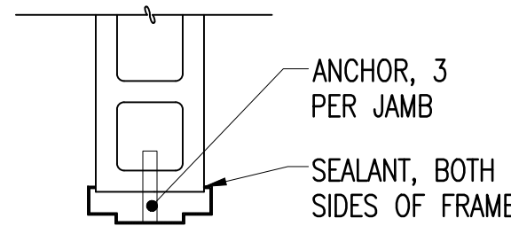
A JAMB
