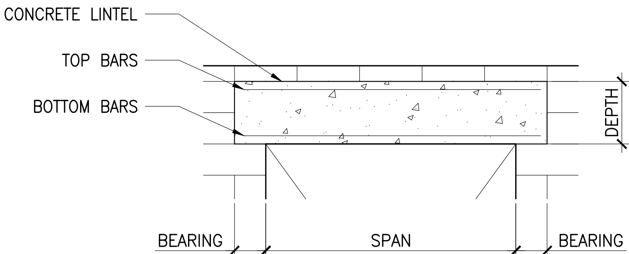
C4 DETAIL SCALE: NTS
