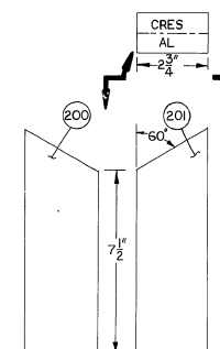
DET 5M-IB DMGT1/GTM200 & GTM201 SCALE: 6'-1-0" (INSTL DET SHTS 3J & 3K)
