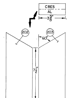
DET 5M-2B DMGT1/GTM202 & GTM203 SCALE: 6'-1-0" (INSTL DET SHTS 3J & 3K)
