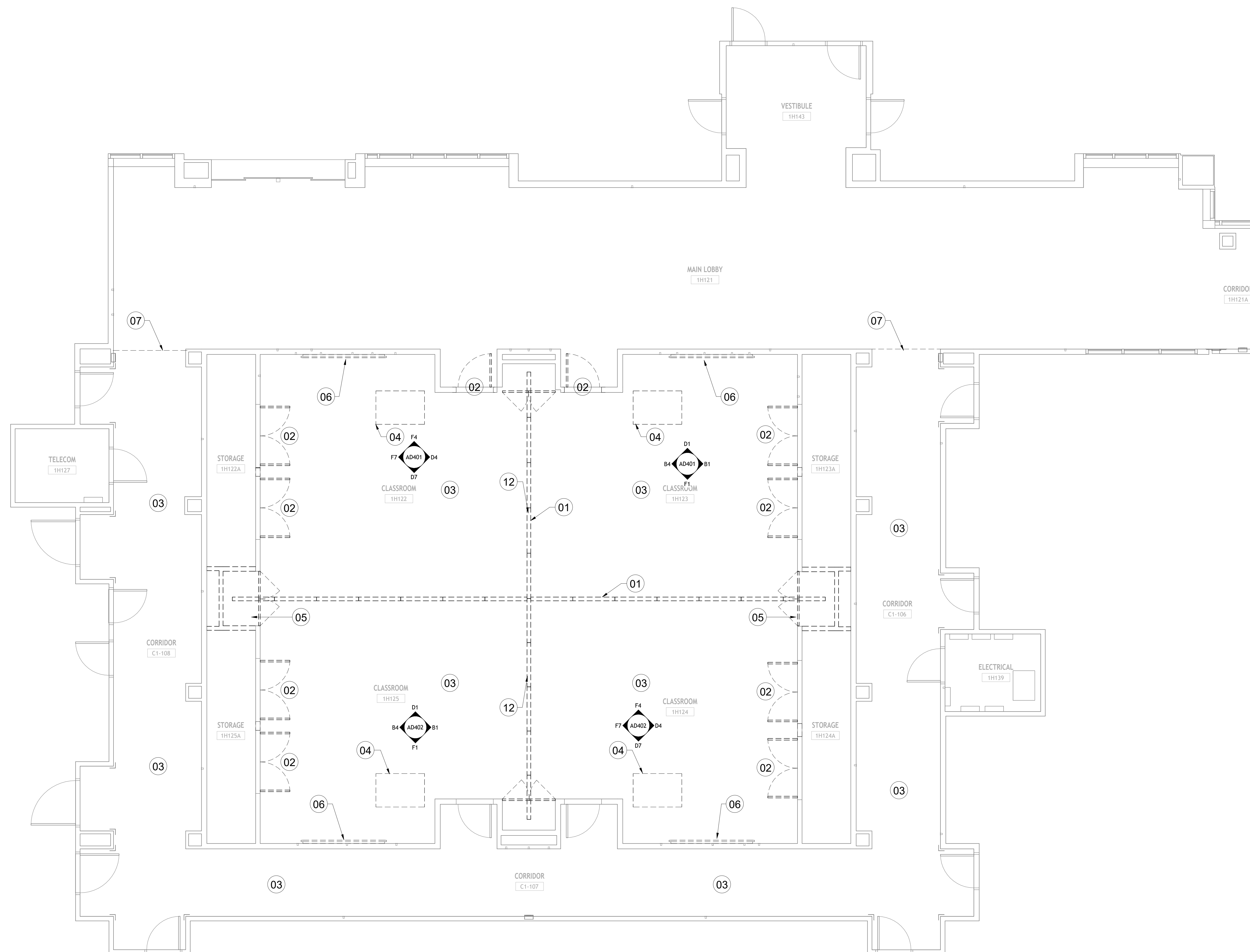
F1 DEMO WORK FLOOR PLAN 1/4" = 1'-0"
