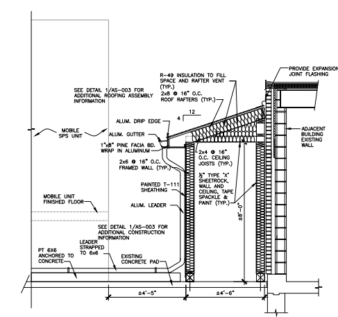
5 CORRIDOR SECTION SCALE: 1/2"=1'-0"
