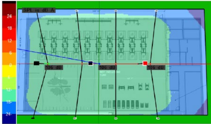
Est. A-weighted SPL "Average Level"
