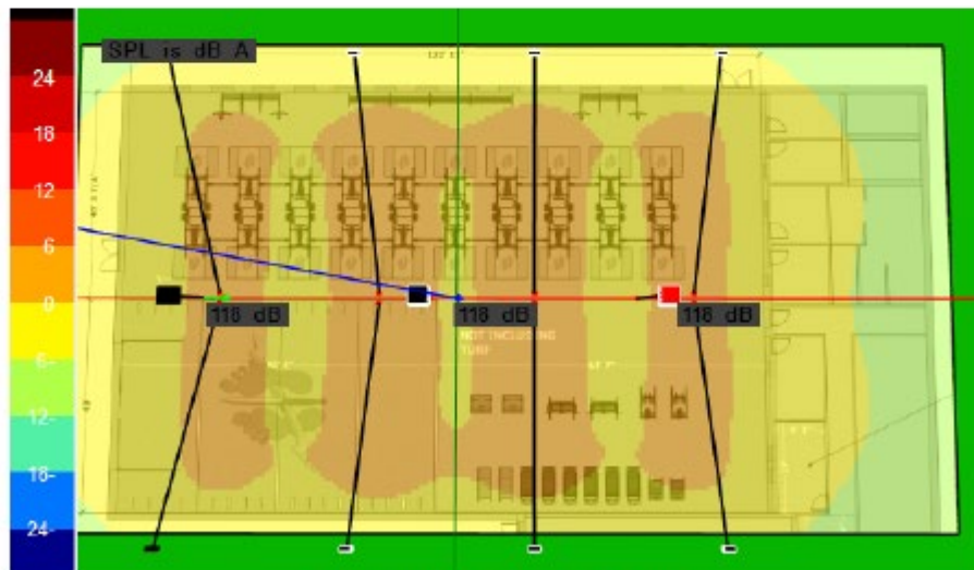
Est. A-weighted SPL "Peak Level"
