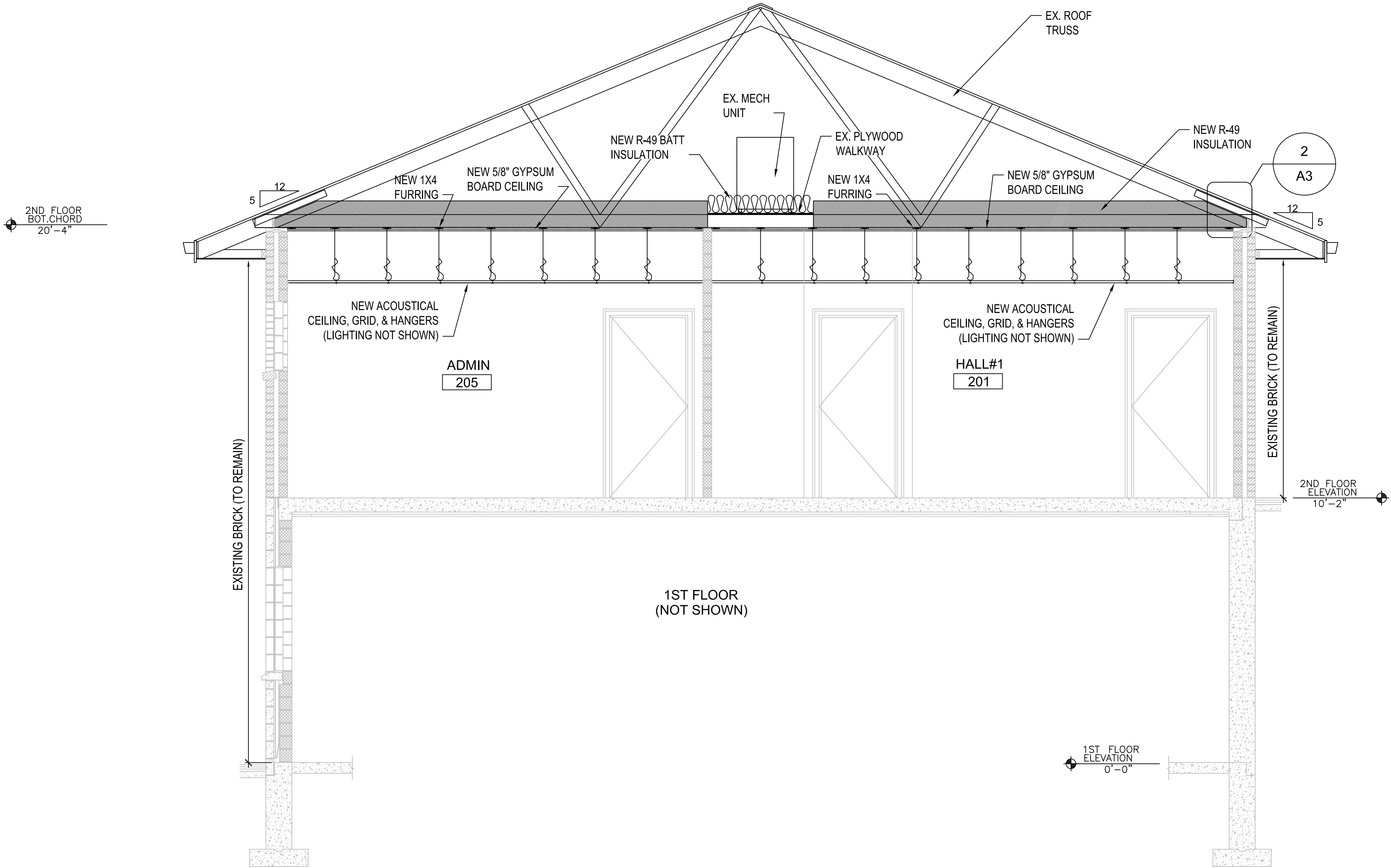
1 SECTION A-A SCALE: 3/8" = 1'-0"
