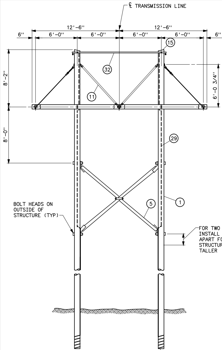
ELEVATION
