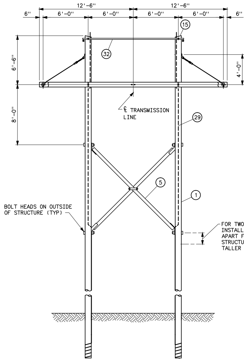
ELEVATION
