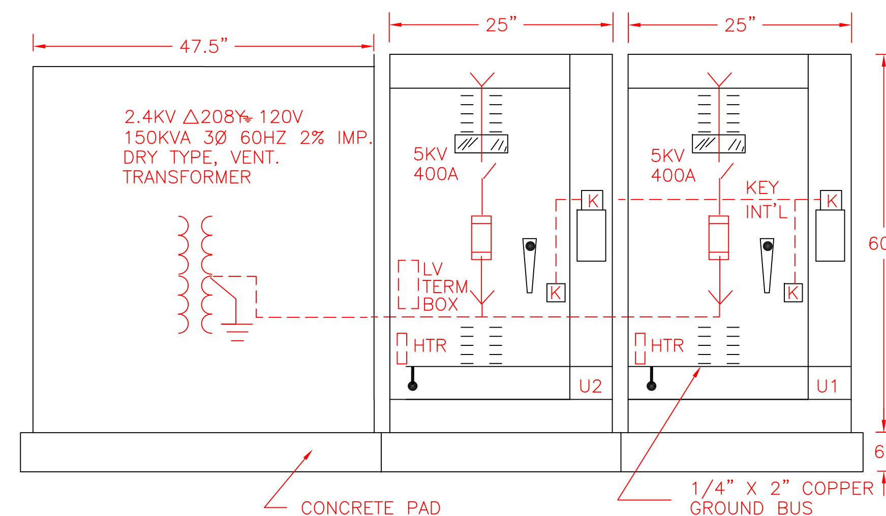
ELEVATION 1/8" = 1'-0" N.T.S.
