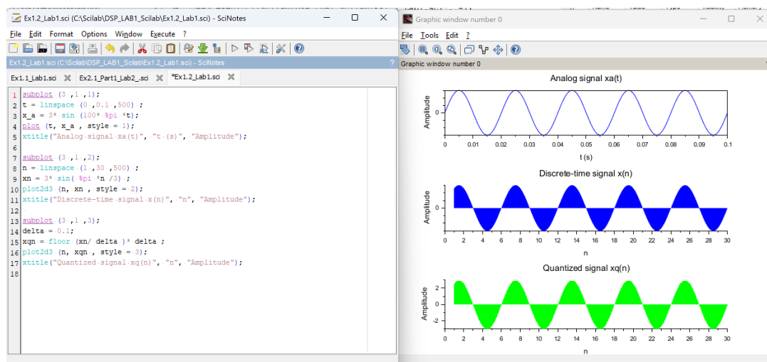
Hình 2: Đồ thị mô phỏng analog signal, discrete-time signal và quantized signal
