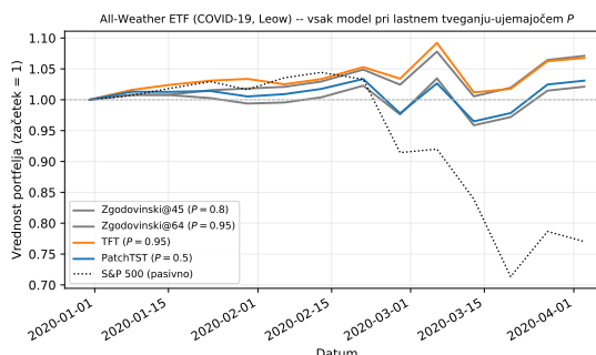
Slika 4. Gibanje vrednosti portfelja All-Weather (5 skladov) skozi zlom ob pandemiji COVID-19 (protokol Leow in sod.). Vsak model je prikazan pri svojem tveganju-ujemajočem P (glej Tabelo 6), tako da so poti neposredno primerljive s poročanimi Sharpovimi količniki; oznake v legendi navajajo uporabljeni P za vsak model. Prikazani so vsi modeli v primerjavi s pasivnim indeksom S&P 500. Vrednosti so bruto, brez transakcijskih stroškov.
