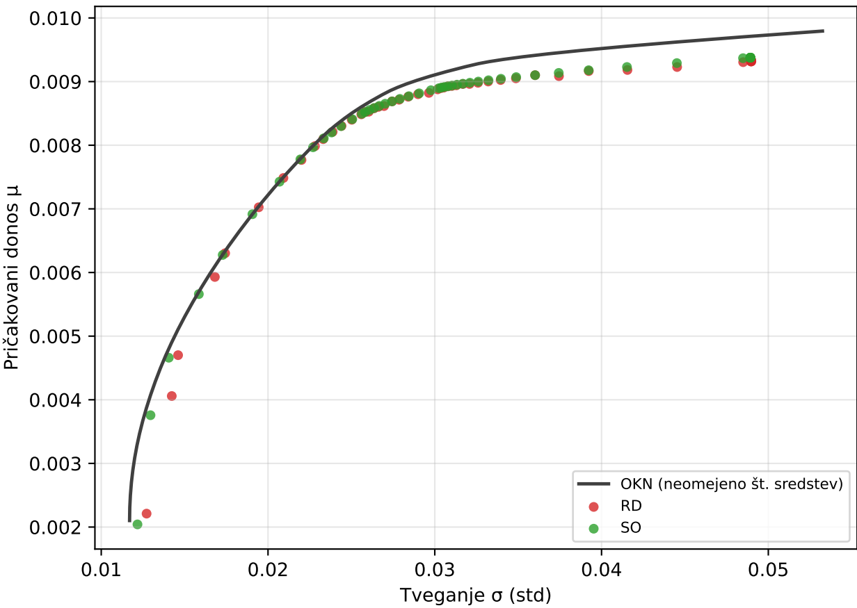
DAX 100 (K=10)
