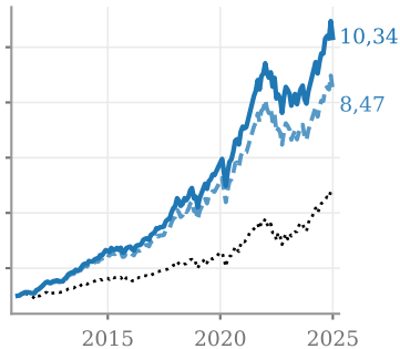
PatchTST + RD
