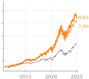
TFT + SO
