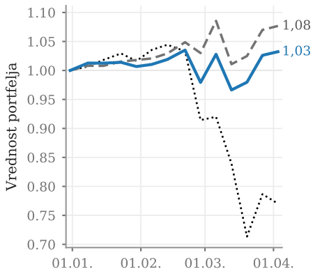
PatchTST + SO / hist. + SO (45 dni)
