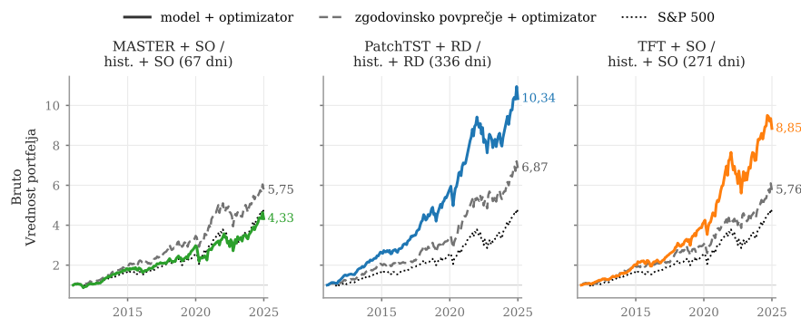
Slika 8. Vrednost portfelja pri dolgoročnem vlaganju (2011–2024), bruto.
