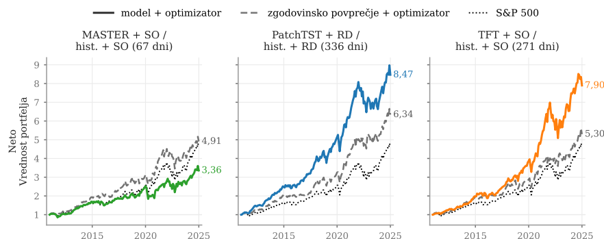
Slika 9. Vrednost portfelja pri dolgoročnem vlaganju (2011–2024), neto.
