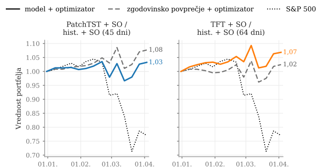
Slika 6. Vrednost portfelja med COVID-19 zlomom: modeli proti zgodovinskemu povprečju.
