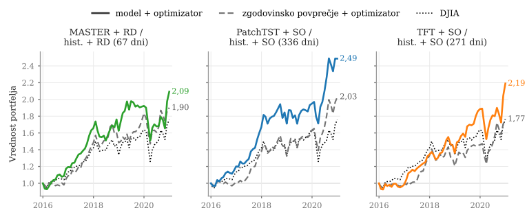
Slika 7. Vrednost portfelja pri mesečnem vlaganju (DJIA, 2016–2020): modeli proti zgodovinskemu povprečju.
