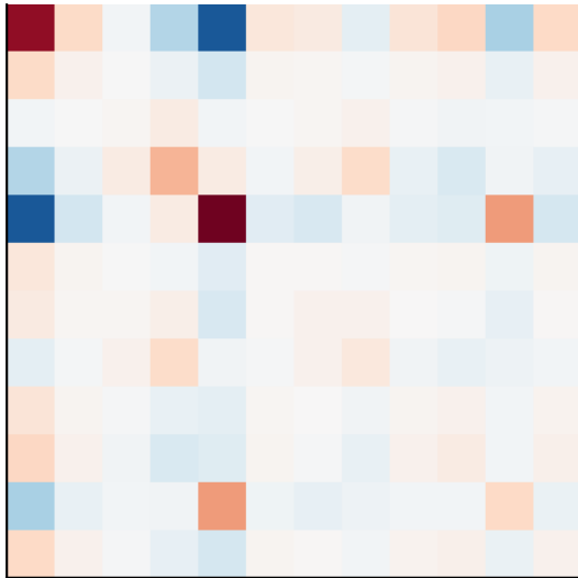
BB^T (nizko-rangno)
