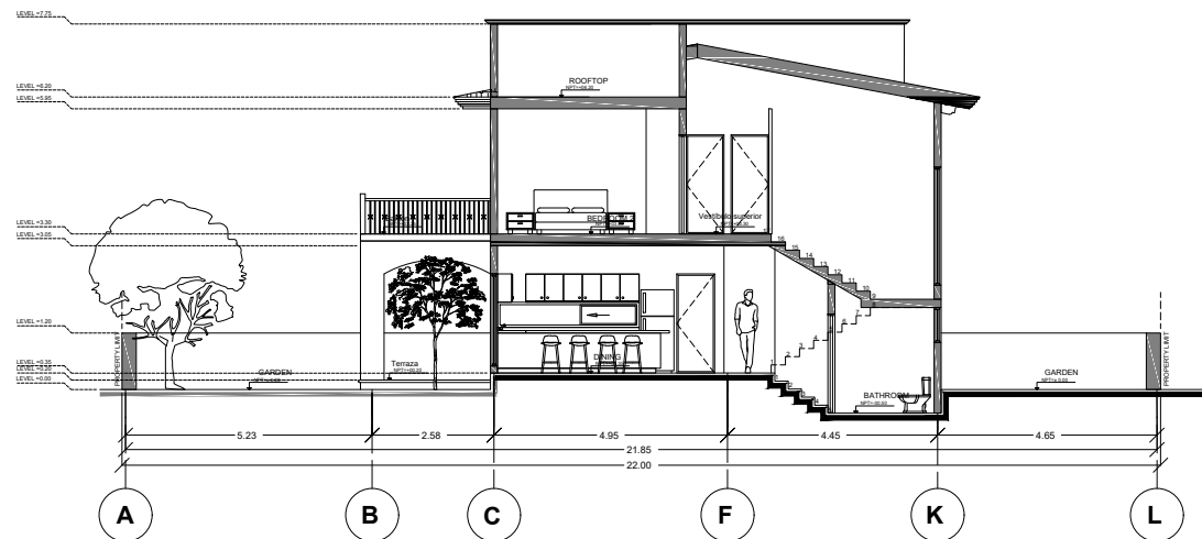
Corte B CASA COLONIAL JAZMIN SCALE 1:50
