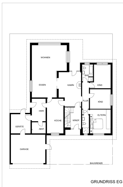
Erdgeschoss · ca. 165,70 m²
