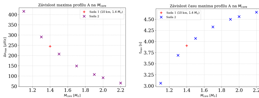
Obrázek 3.16. Závislost maxima a času maxima profilu A na hmotnosti M_{core} .
