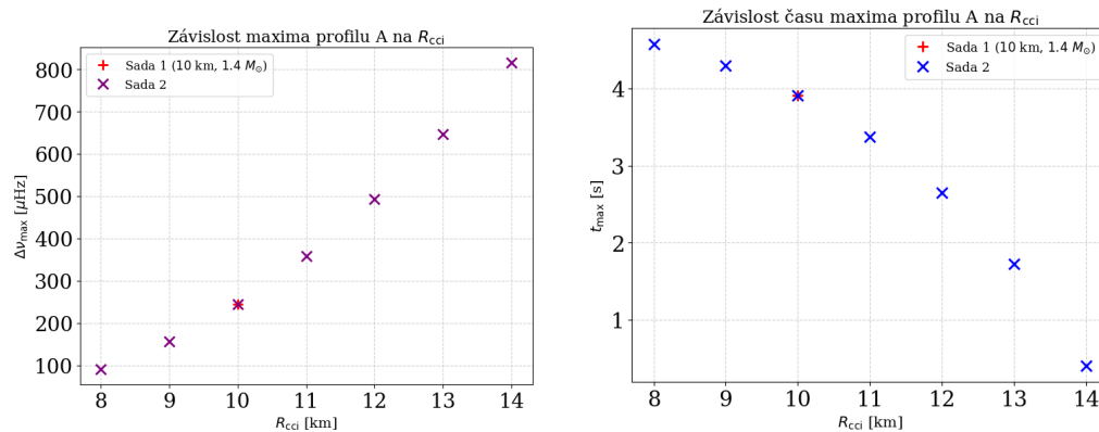
Obrázek 3.15. Závislost maxima a času maxima profilu A na poloměru rozhraní R_{cci} .
