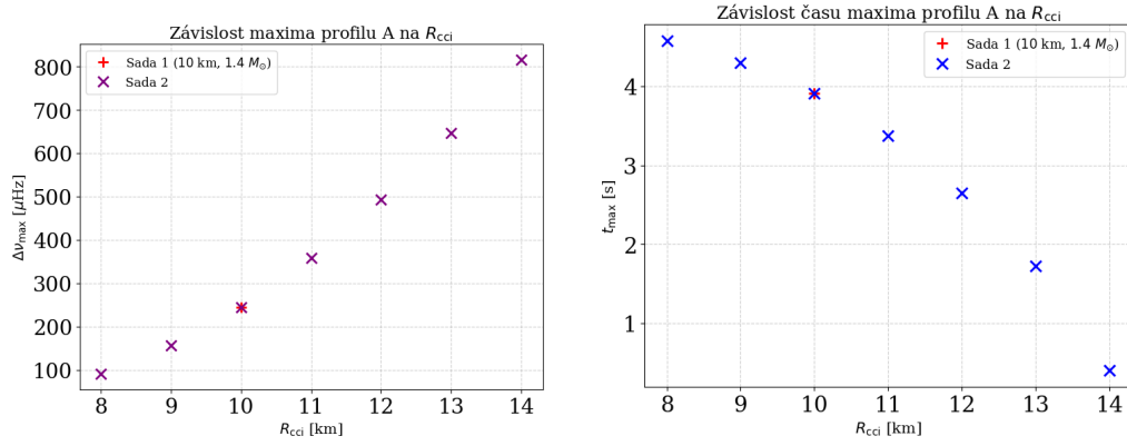
Obrázek 3.16. Závislost maxima a času maxima profilu A na poloměru rozhraní R_{cci} .
