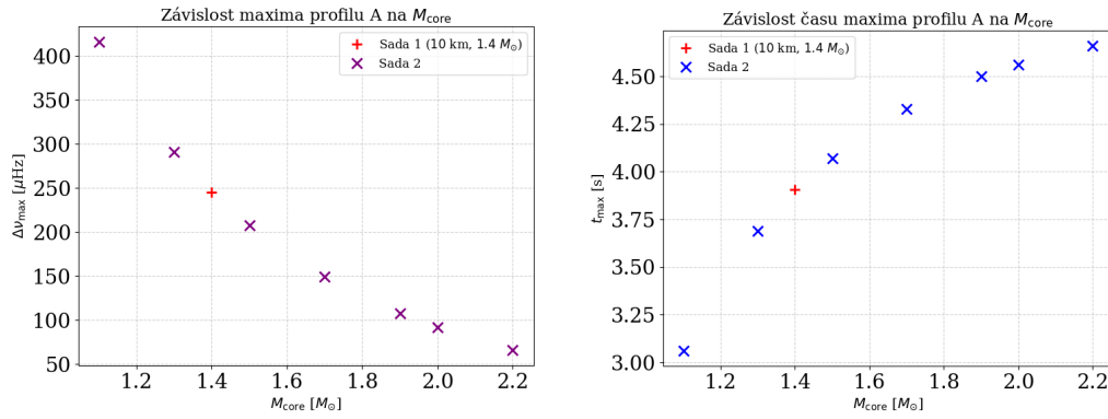
Obrázek 3.17. Závislost maxima a času maxima profilu A na hmotnosti M_{core} .
