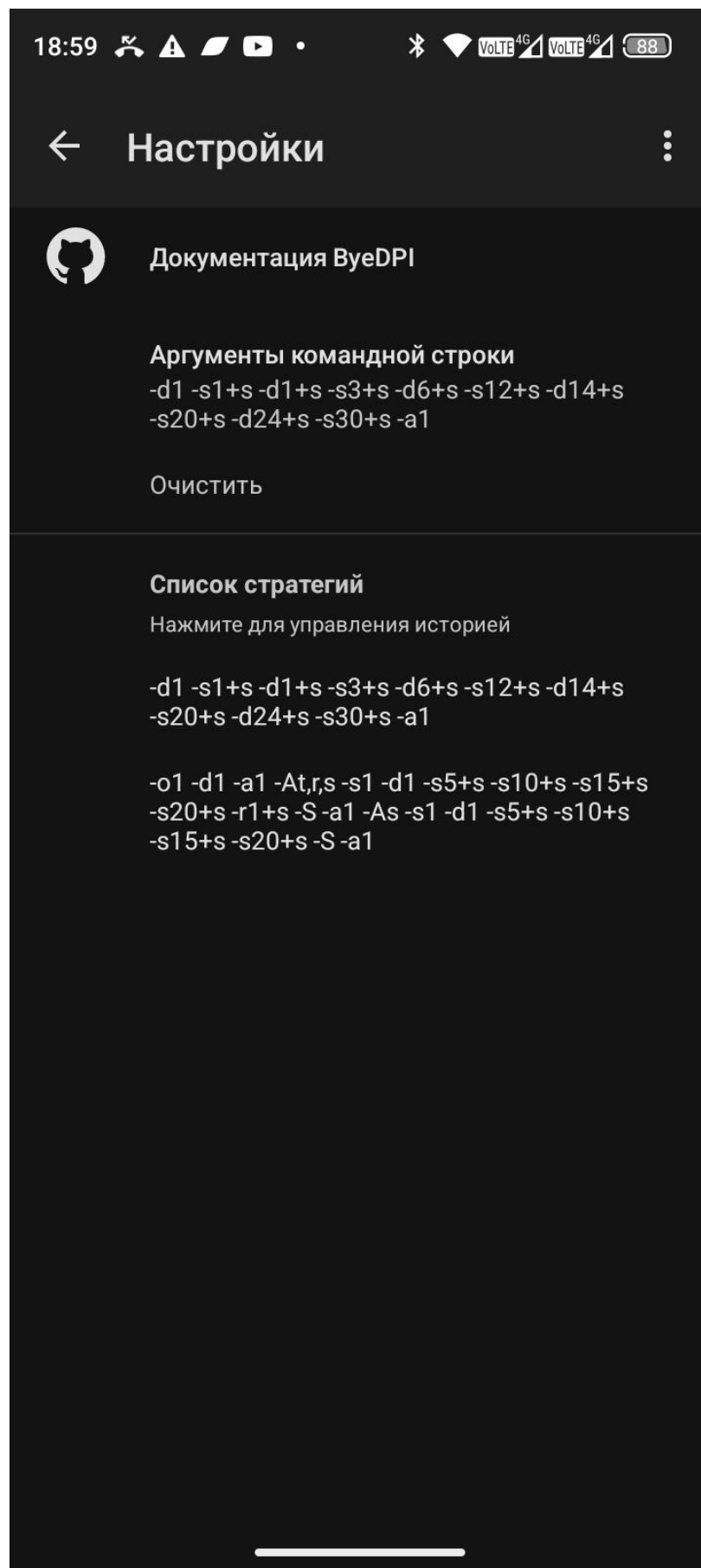
Рисунок 3 – Редактор командной строки
