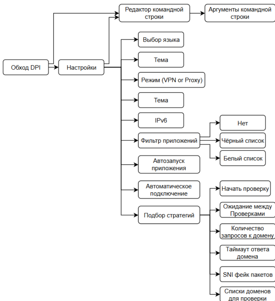
Рисунок 7 – Реализация Mind Map
