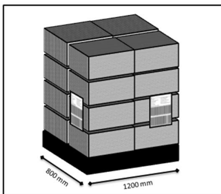
Figura 16 – Colocação de Etiqueta GS1-128 / EAN128 em Paletes mono-referência
