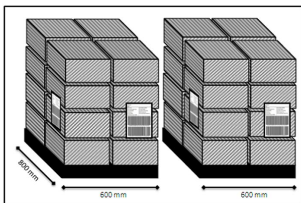
Figura 19 – Identificação GS1-128 / EAN 128 em ½ Paletes PBL
