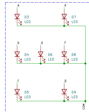
Dobbelsteen Alle LEDs 2mA type, in kleur naar keuze
