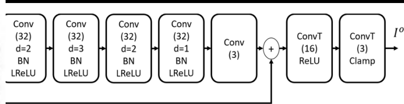
CNN-deblurring network
