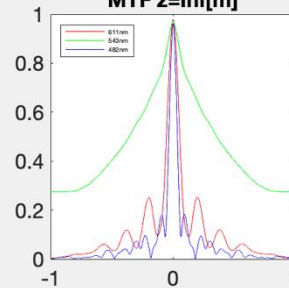
MTF z=Inf[m]
