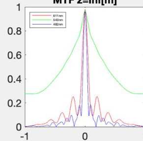
MTF z=Inf[m]
