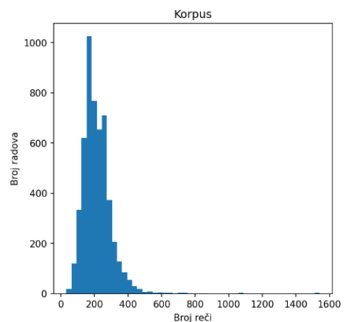
Slika III.1 Histogram dužine radova
