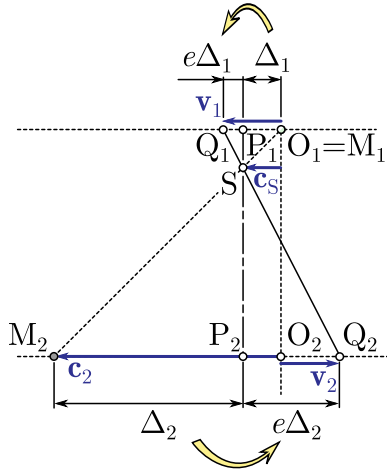
7. ábra: Az ütközés Maxwell-ábrája
