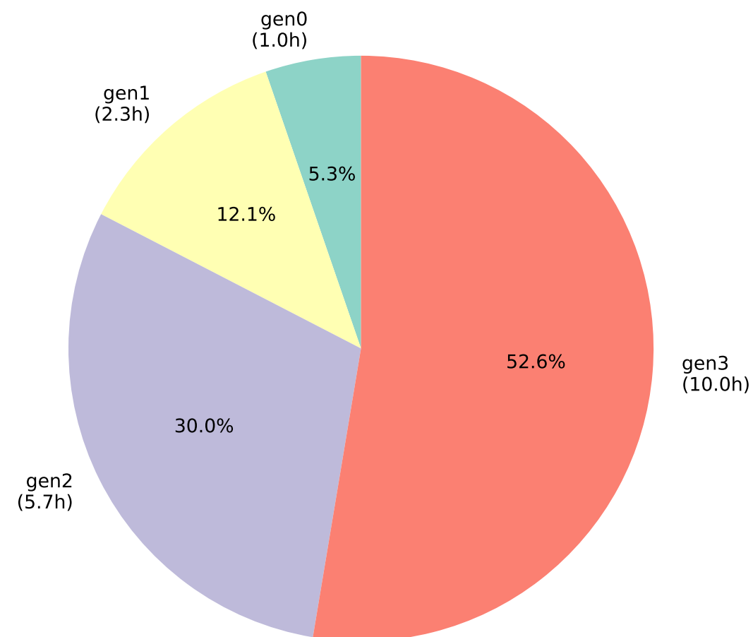
NanoMQ ASE Distribution (Total Fuzz: 19.0h)
