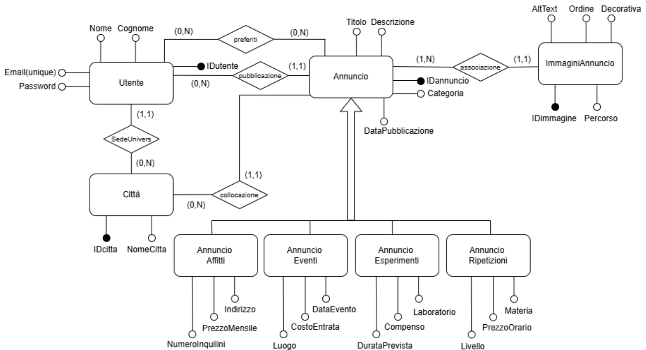
Figura 2: Schema ER
