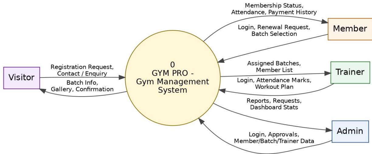
Fig 4.2(a): DFD Level 0 (Context Diagram)
