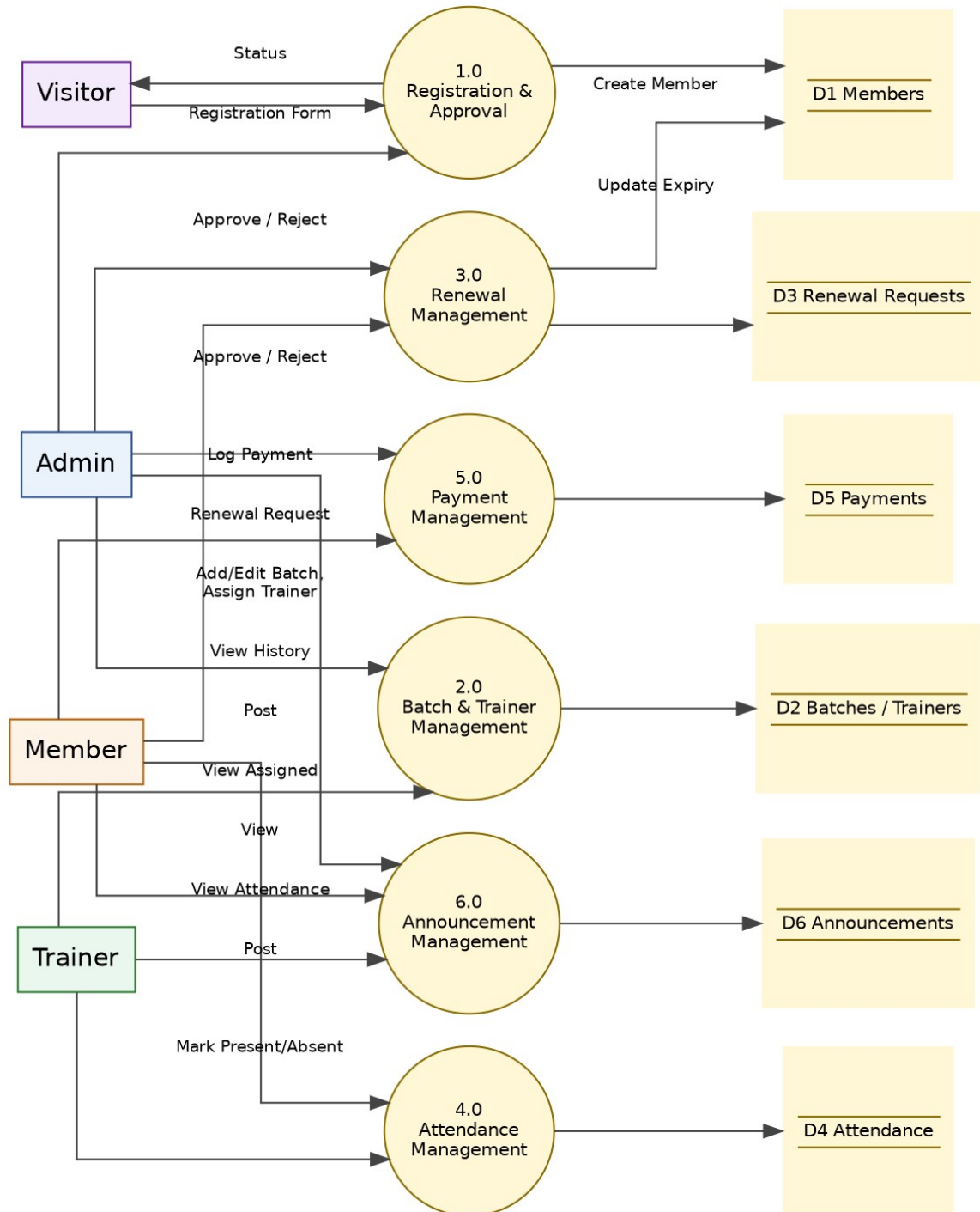
Fig 4.2(b): DFD Level 1
