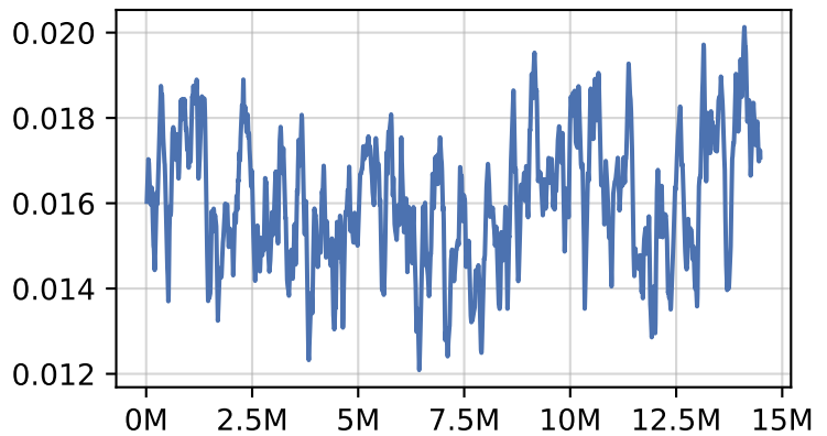
MortarMayhem-v0
