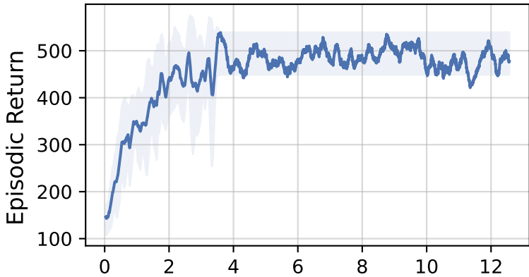
Humanoid-v4
