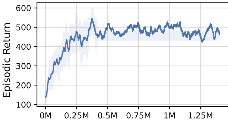
Humanoid-v4
