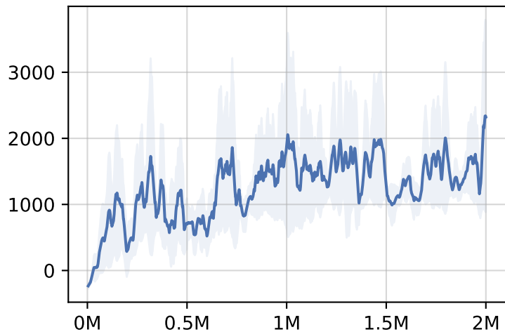
Humanoid-v4
