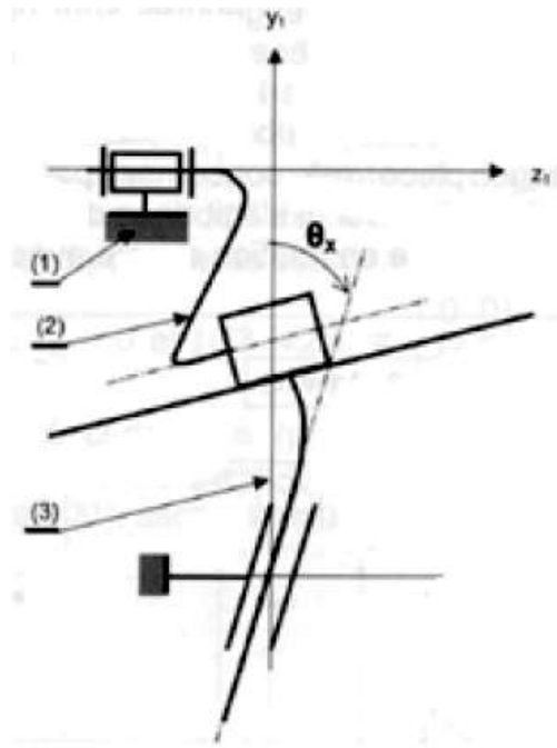
Figure 5 – Influence du défaut \theta_x
