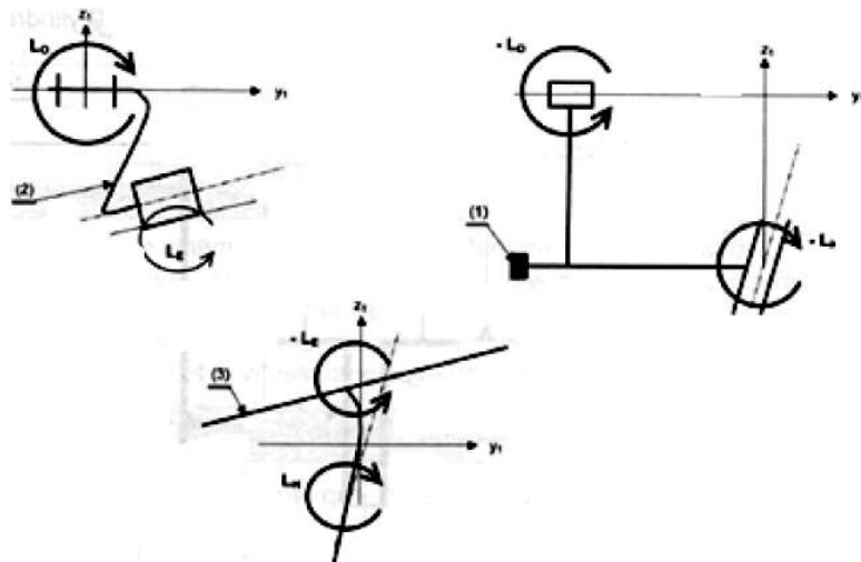
Figure 6 – Inconnues de liaison L_i
