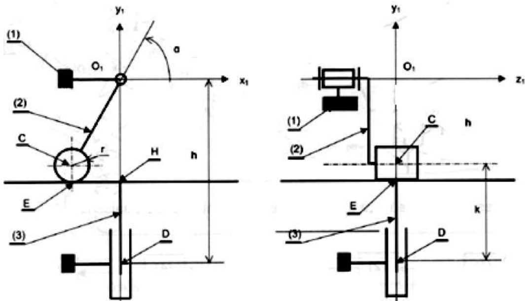
Figure 3 – Paramétrage (vues de face et de gauche)
