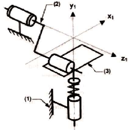
Figure 2 – Schéma cinématique
