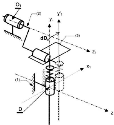
Figure 11 – Défaut dD_x en D
