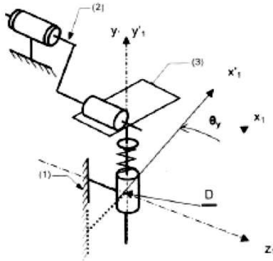
Figure 8 – Défaut \theta_y en D
