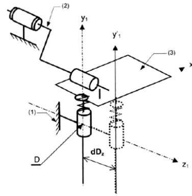
Figure 12 – Défaut dD_z en D
