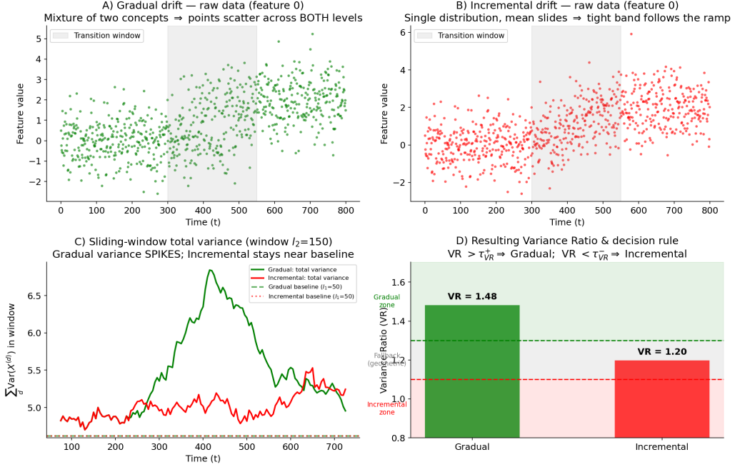
Hình 4.6 Minh hoạ cơ chế Variance Ratio (VR) trên dữ liệu thô. (A, B) Dữ liệu thô của Gradual và Incremental drift: hỗn hợp xác suất làm dữ liệu Gradual trải trên hai mức, còn Incremental là một dải hẹp trượt dần. (C) Phương sai trên cửa sổ trượt: Gradual nhô lên trên baseline (do thành phần between-concept theo Eq. (4.5)), Incremental giữ gần baseline. (D) Giá trị VR thu được và vùng quyết định: VR > \tau_{VR}^+ \Rightarrow \text{Gradual} ; VR < \tau_{VR}^- \Rightarrow \text{Incremental} ; vùng giữa lùi về quy tắc hình học.
