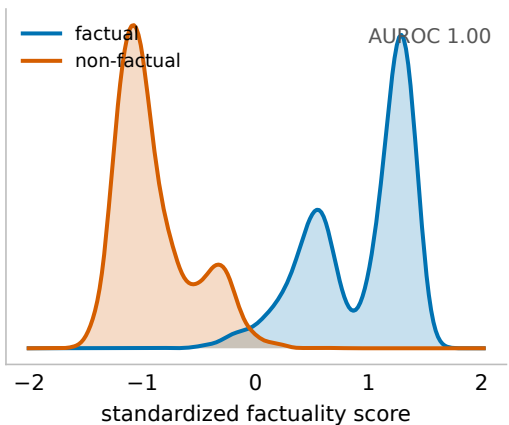
Internal score — Llama-3.1-8B
