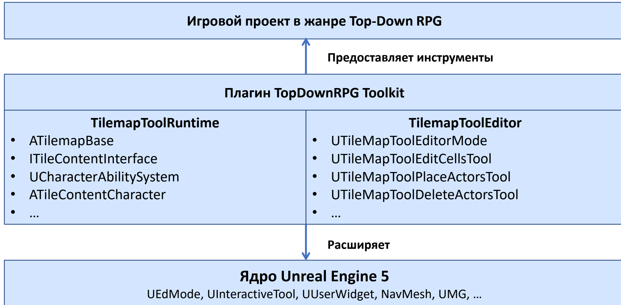
Рисунок 2 – Архитектура проекта
