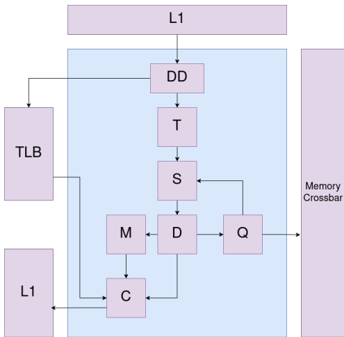
Рис. 2: Партиция L2 кэша GPGPU.
