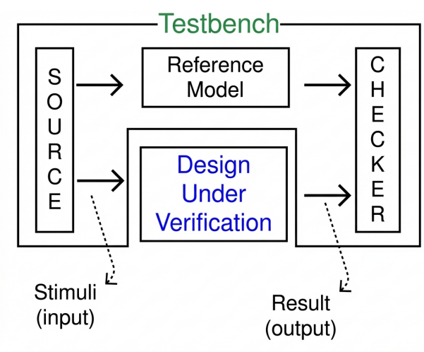
Рис. 1: Структура тестбенча.
