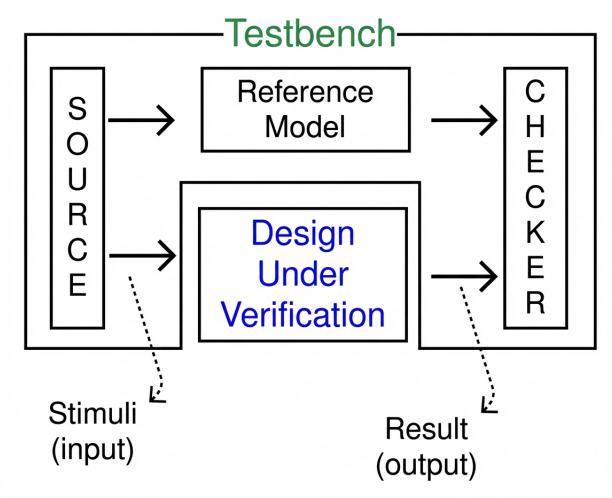
Рис. 1: Структура тестбенча.
