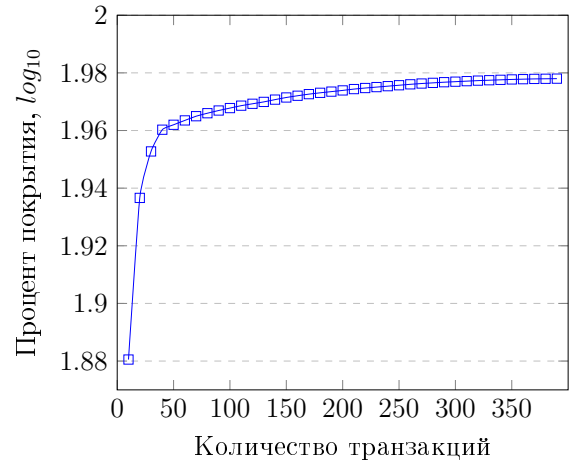
Рис. 14: Процент кодового покрытия в зависимости от количества транзакций в логарифмическом масштабе для Q-stage.
