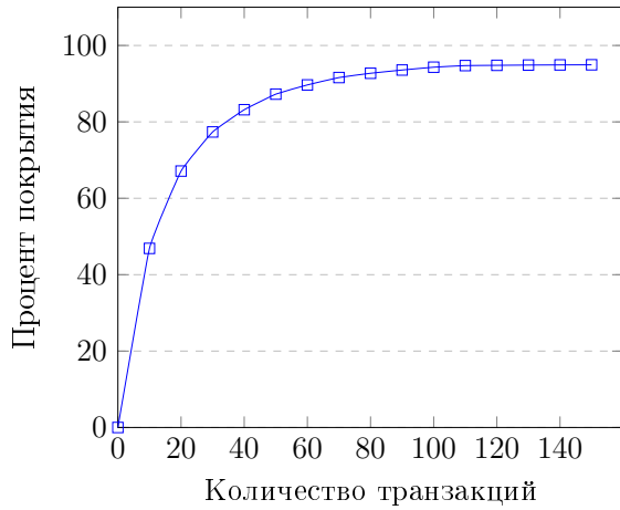
Рис. 7: Процент кодового покрытия в зависимости от количества транзакций для C-stage
