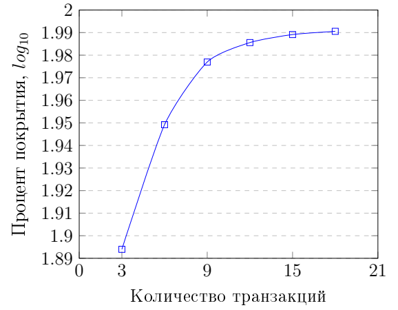
Рис. 10: Процент кодового покрытия в зависимости от количества транзакций в логарифмическом масштабе для DD-stage
