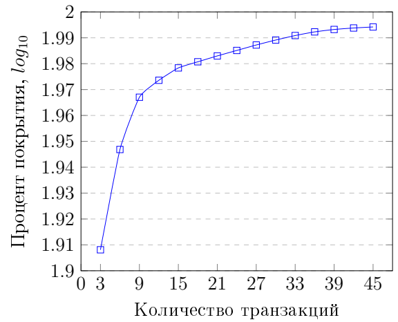
Рис. 6: Процент кодового покрытия в зависимости от количества транзакций в логарифмическом масштабе для D-stage
