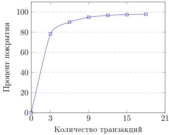
Рис. 9: Процент кодового покрытия в зависимости от количества транзакций для DD-stage
