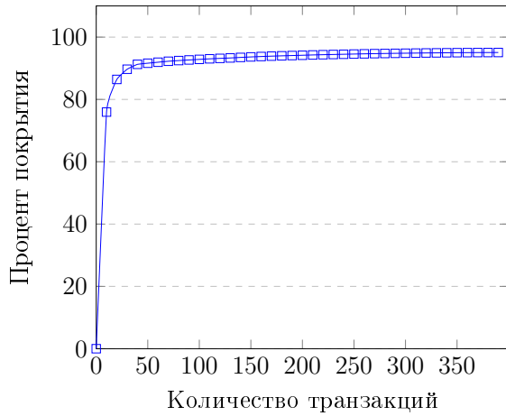
Рис. 13: Процент кодового покрытия в зависимости от количества транзакций для Q-stage.
