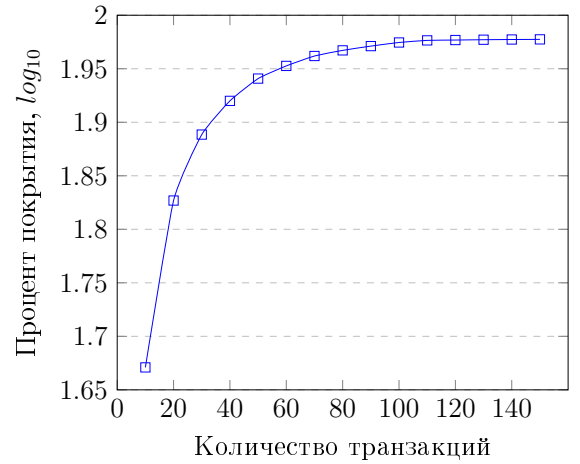
Рис. 8: Процент кодового покрытия в зависимости от количества транзакций в логарифмическом масштабе для C-stage
