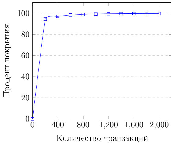
Рис. 11: Процент кодового покрытия в зависимости от количества транзакций для T-stage
