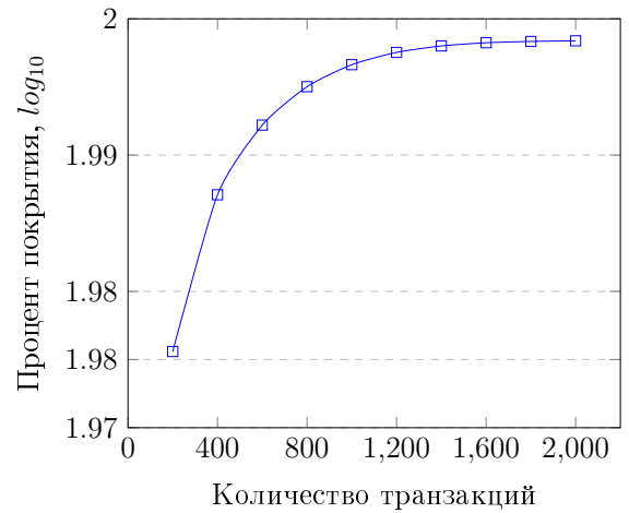
Рис. 12: Процент кодового покрытия в зависимости от количества транзакций в логарифмическом масштабе для T-stage
