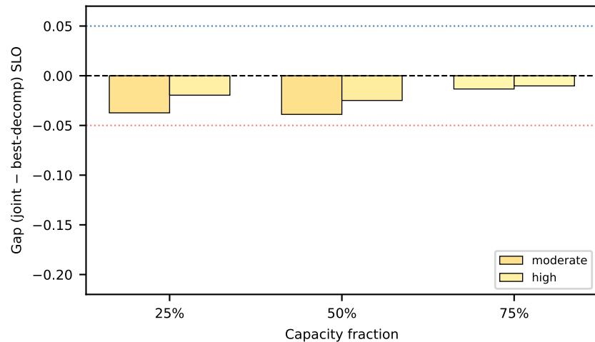
tau=0.95, mostly_dense
